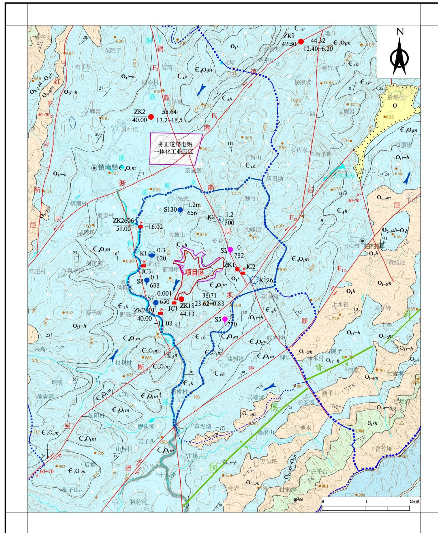
图 4.3-7 调查评价区 1:5 万水文地质图
