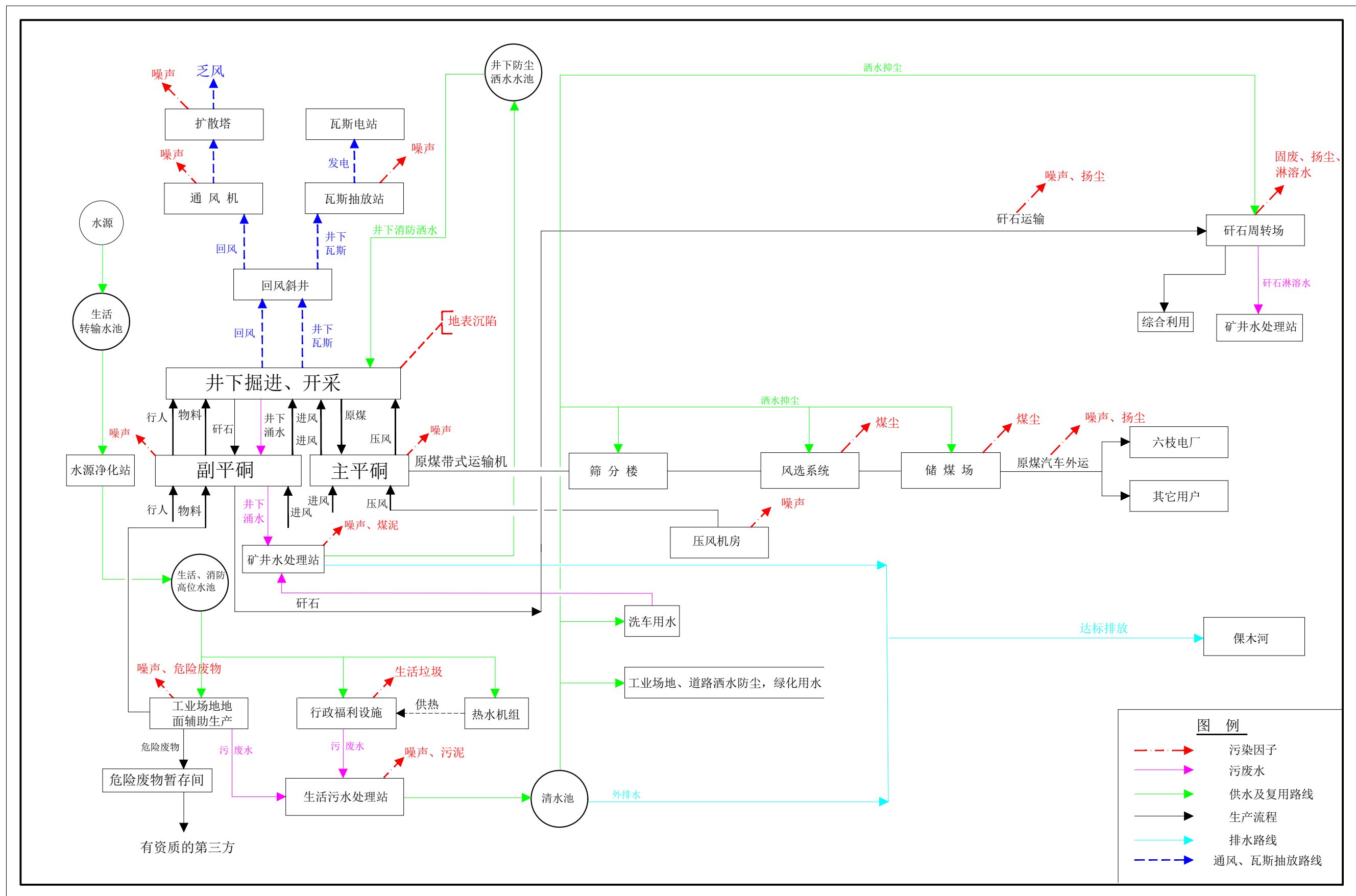
图3.4-1 六家坝煤矿（兼并重组）生产流程及污染物产生环节示意图
