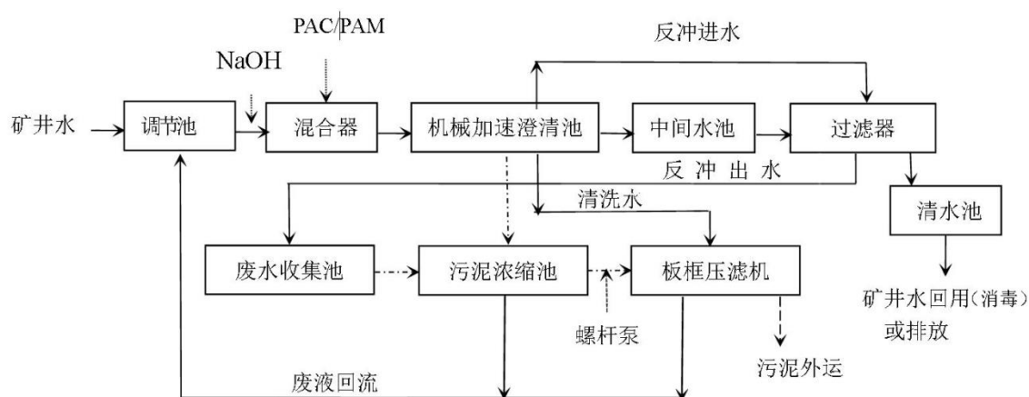
图 7.5-1 六家坝煤矿矿井水处理工艺流程图
