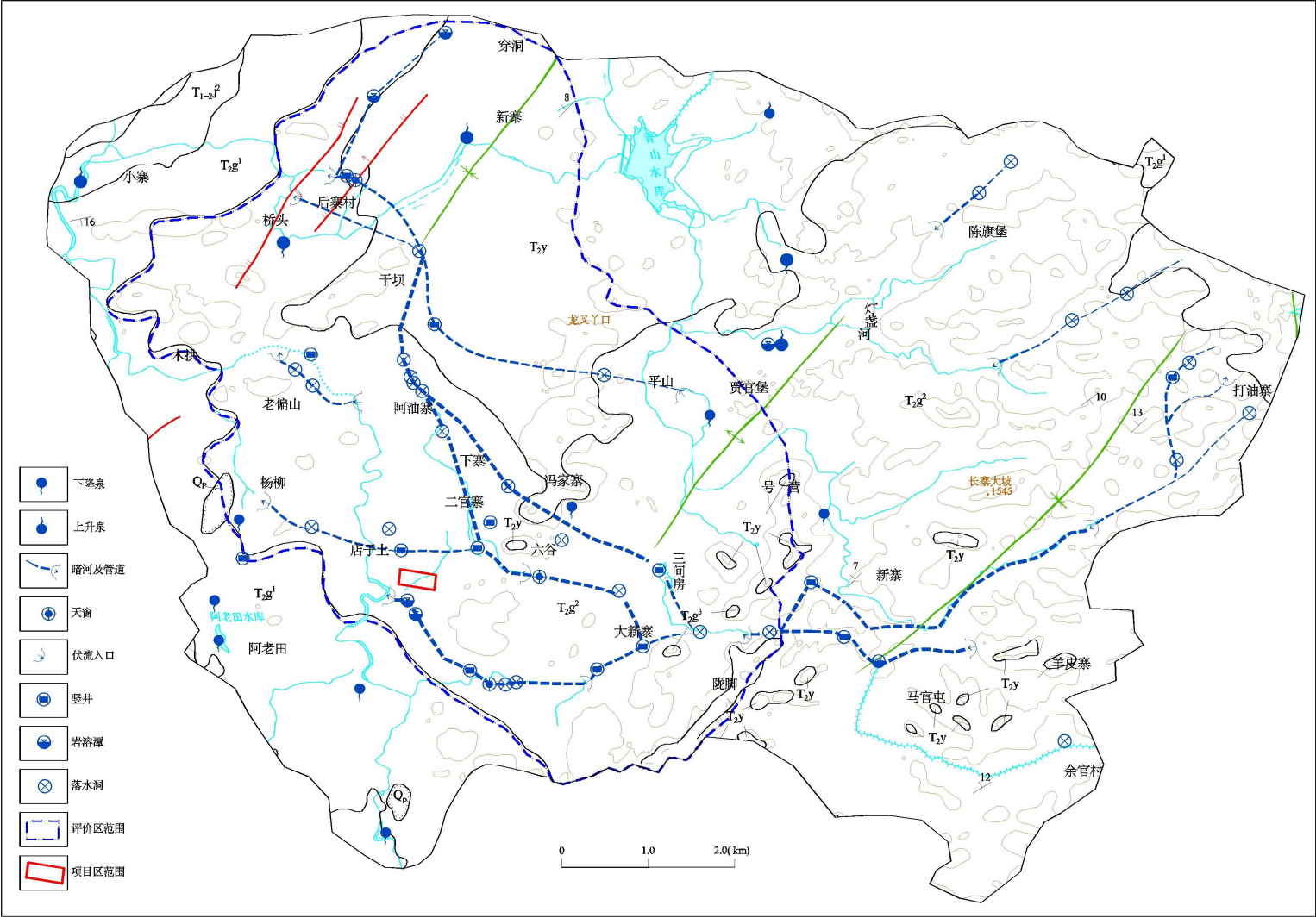
图 5.4-5 后寨地下河系统-母猪洞支流及水洞支流下游次系统平面示意图
