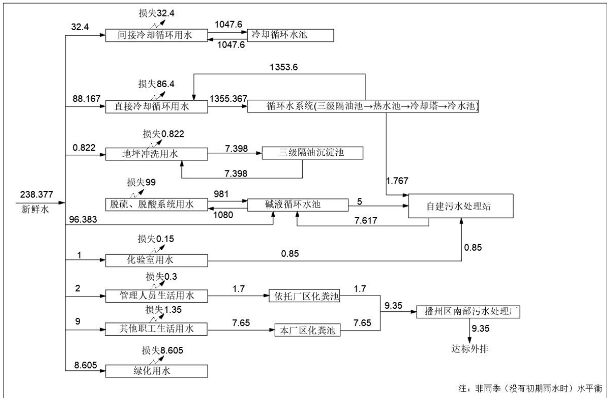
图 3.1-2 非雨季项目全厂水平衡图（单位：m³/d）
