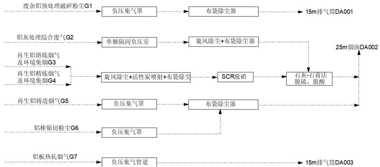
图 3.4-1 本项目废气污染防治及排放系统图
