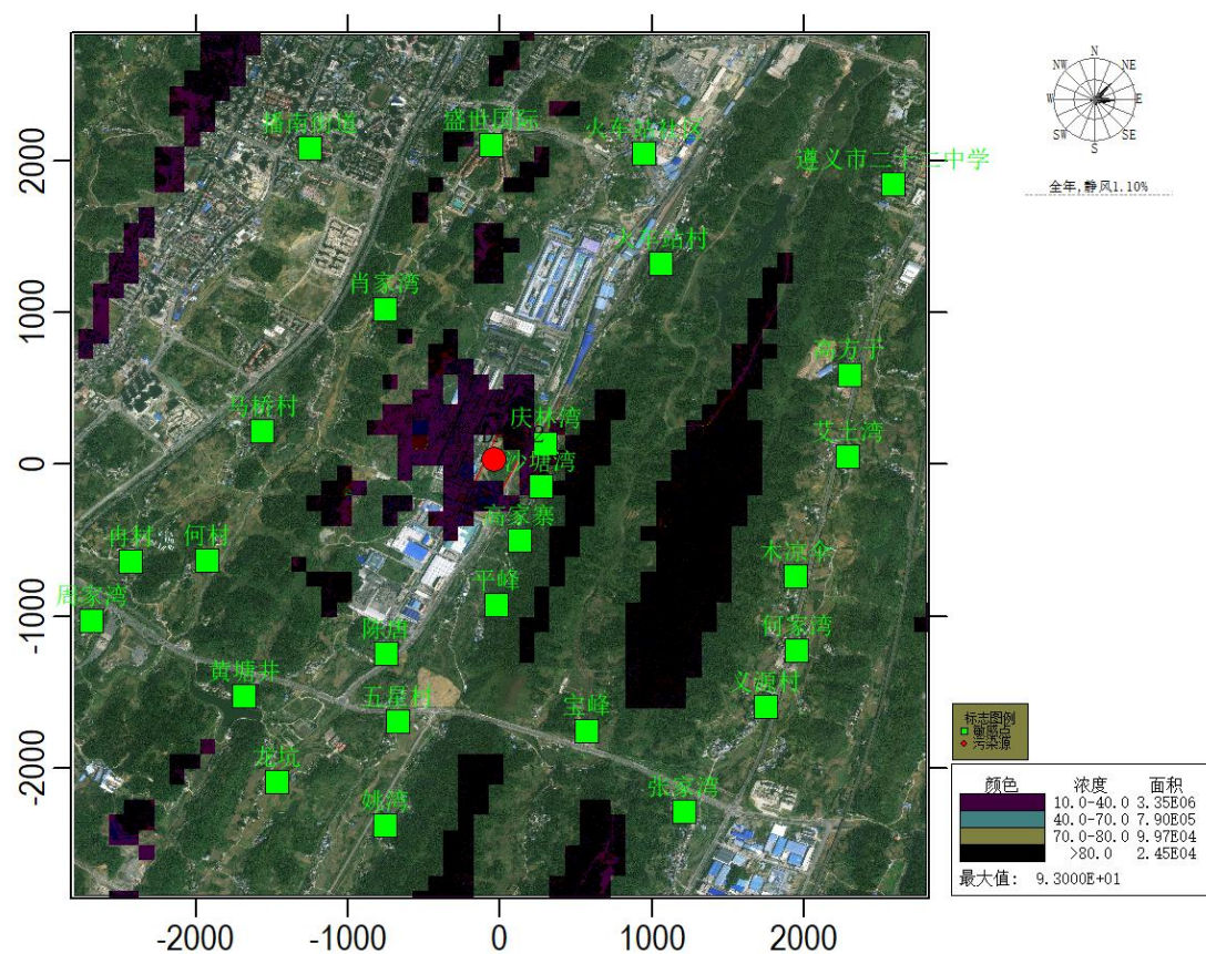
图 5.4.3-22 非正常工况下氟化物 1h 平均质量浓度分布图 (单位: \mu\text{g}/\text{m}^3 )
