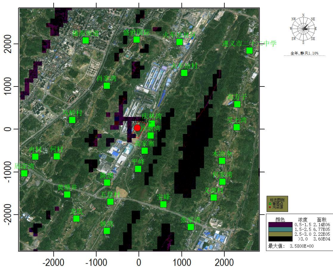
图 5.4.3-21 非正常工况下 HCl1h 平均质量浓度分布图 (单位: \mu g/m^3 )
