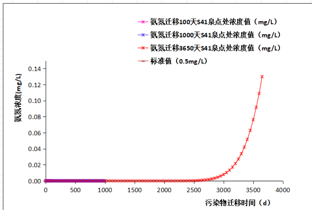
图 5.3.2-10 非正常状况下污染物氨氮向南侧 S41 号泉点处迁移不同时间浓度曲线图
