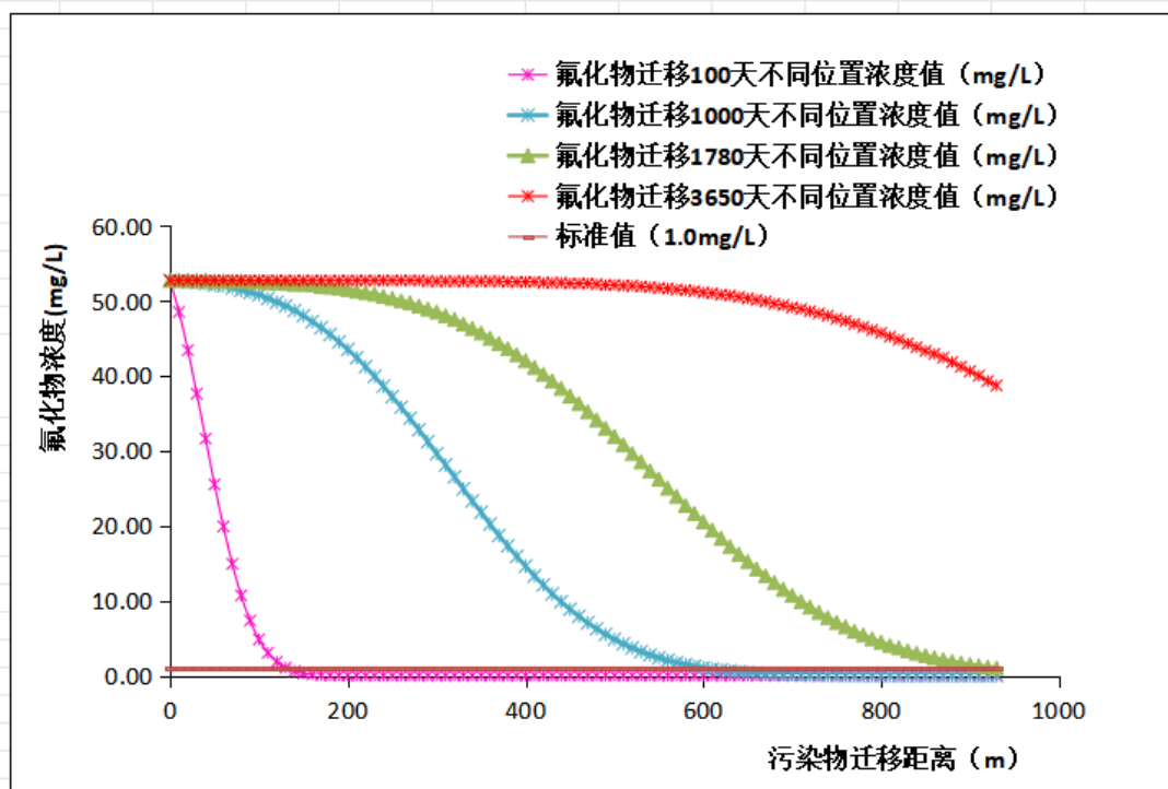
图 5.3.2-1 非正常状况下污染物氟化物向南西侧迁移不同时间不同位置距离浓度曲线图
