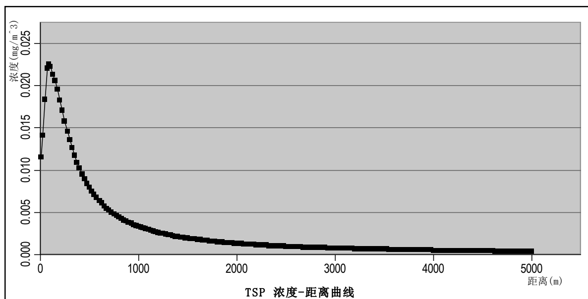
图 5.2.2-1 TSP 占标率——距离曲线图
