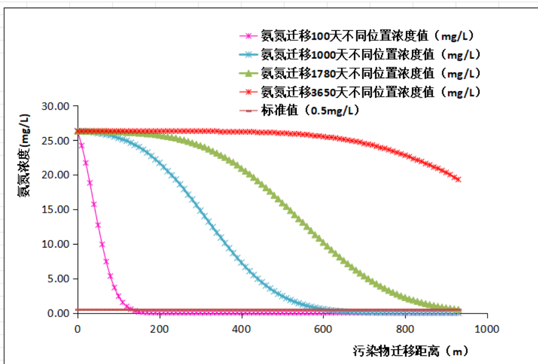
图 5.3.2-3 非正常状况下污染物氨氮向南侧迁移不同时间不同位置距离浓度曲线图
