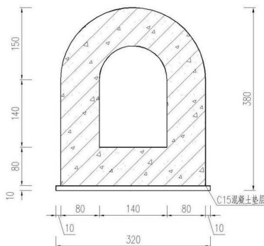
图 2.4.3-2 排水箱涵结构断面图
