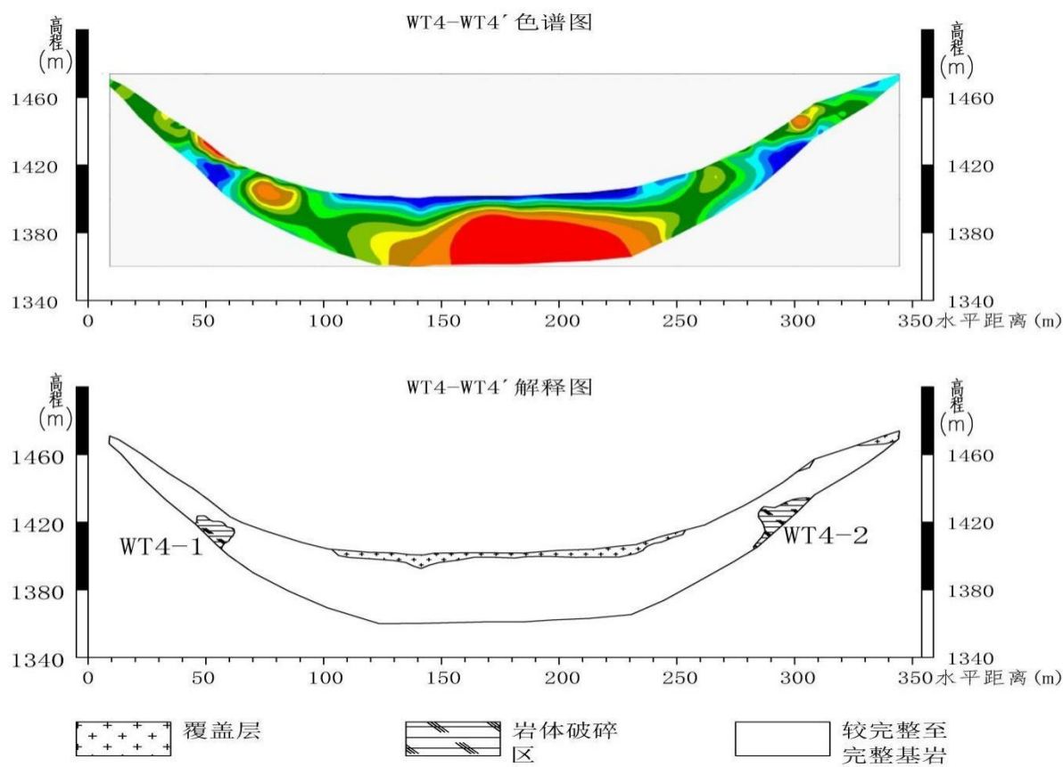
图 4.2.3-4 库盆内高密度电法测试异常解译图
