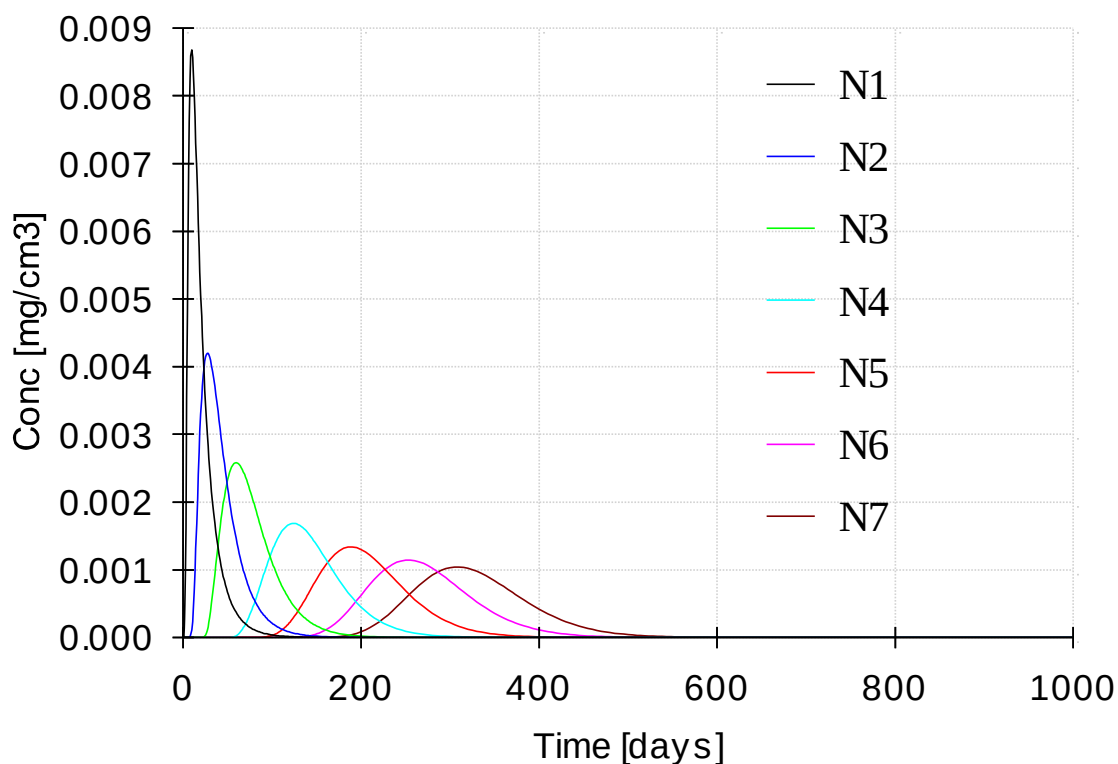
图 5.7-3 当发生废水短时间渗漏 3d 时氟化物土壤污染预测图
