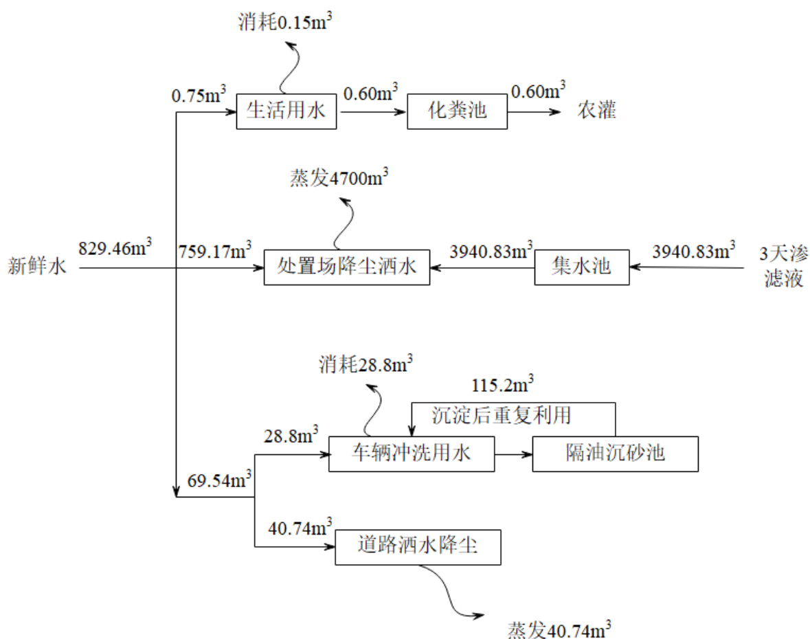
图 3.3-3 本工程营运期水平衡图 (3 天)
