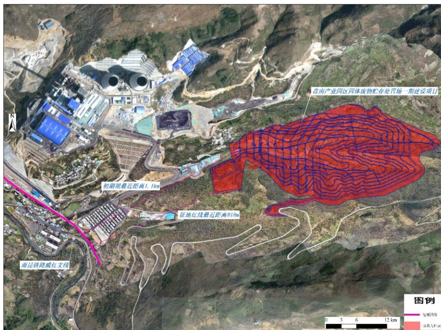
图 3.2-2 本工程与南昆铁路威红支线区位关系图
