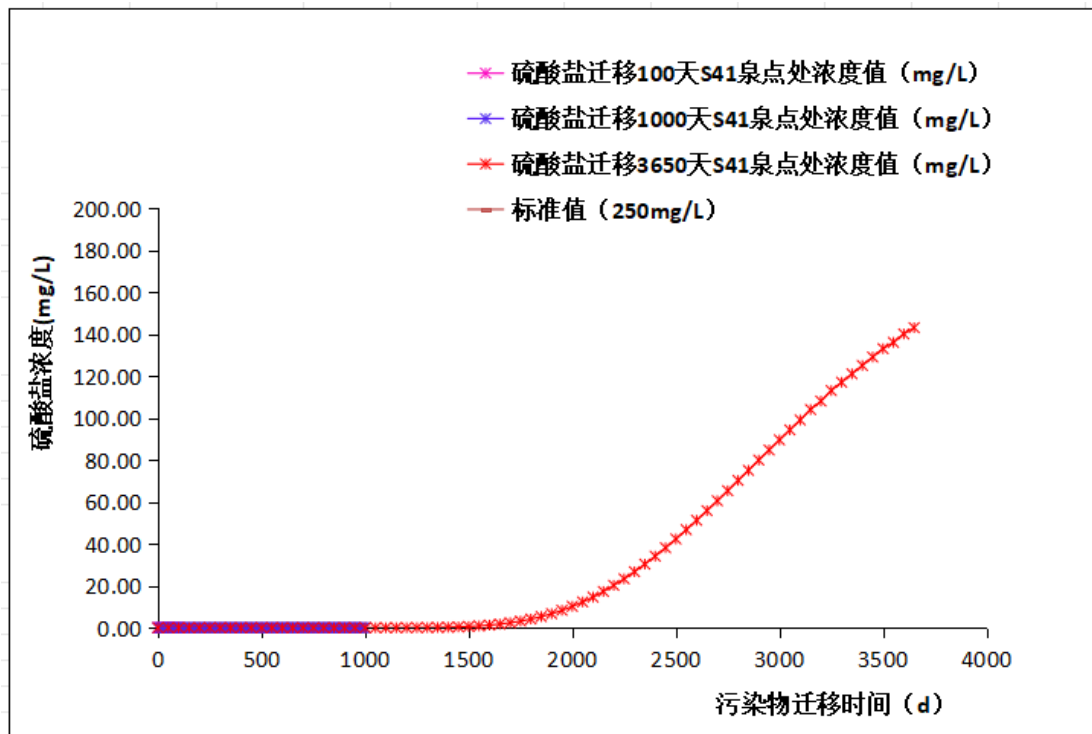
图 5.3.2-6 非正常状况下污染物硫酸盐向南侧 S41 号泉点处迁移不同时间浓度曲线图
