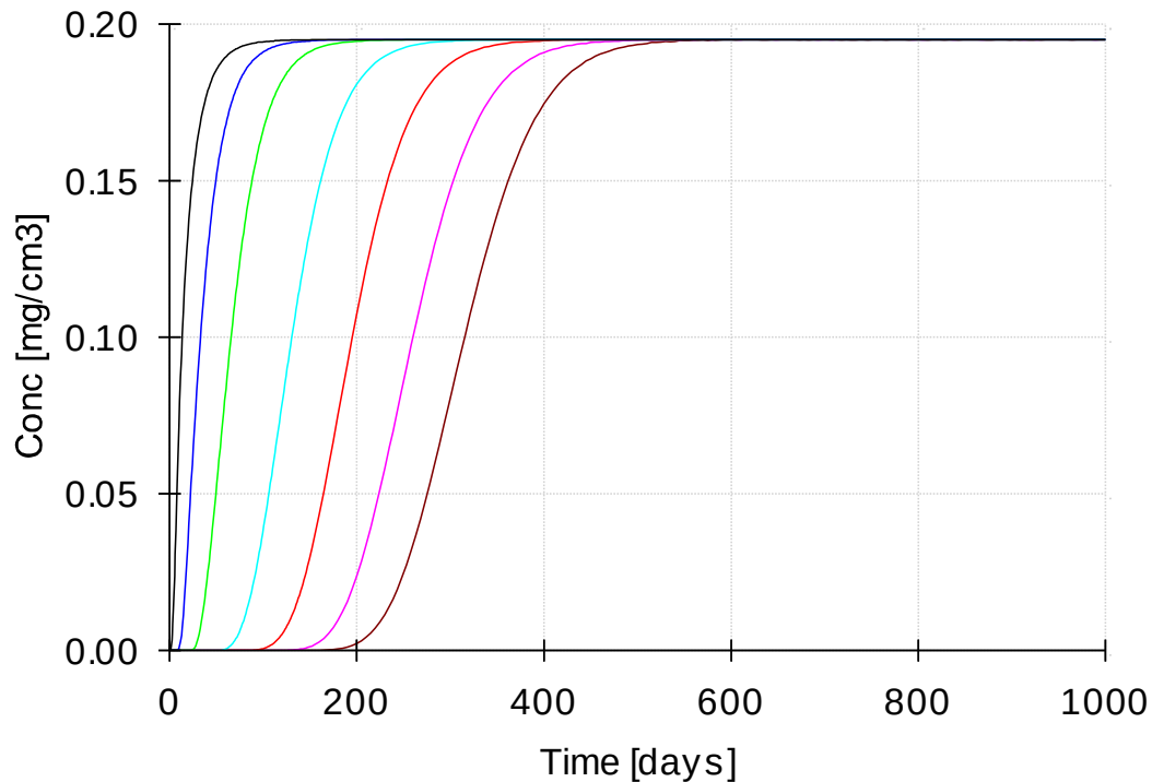
图 5.7-2 当发生废水持续渗漏 1000d 时硫酸盐土壤污染预测图
