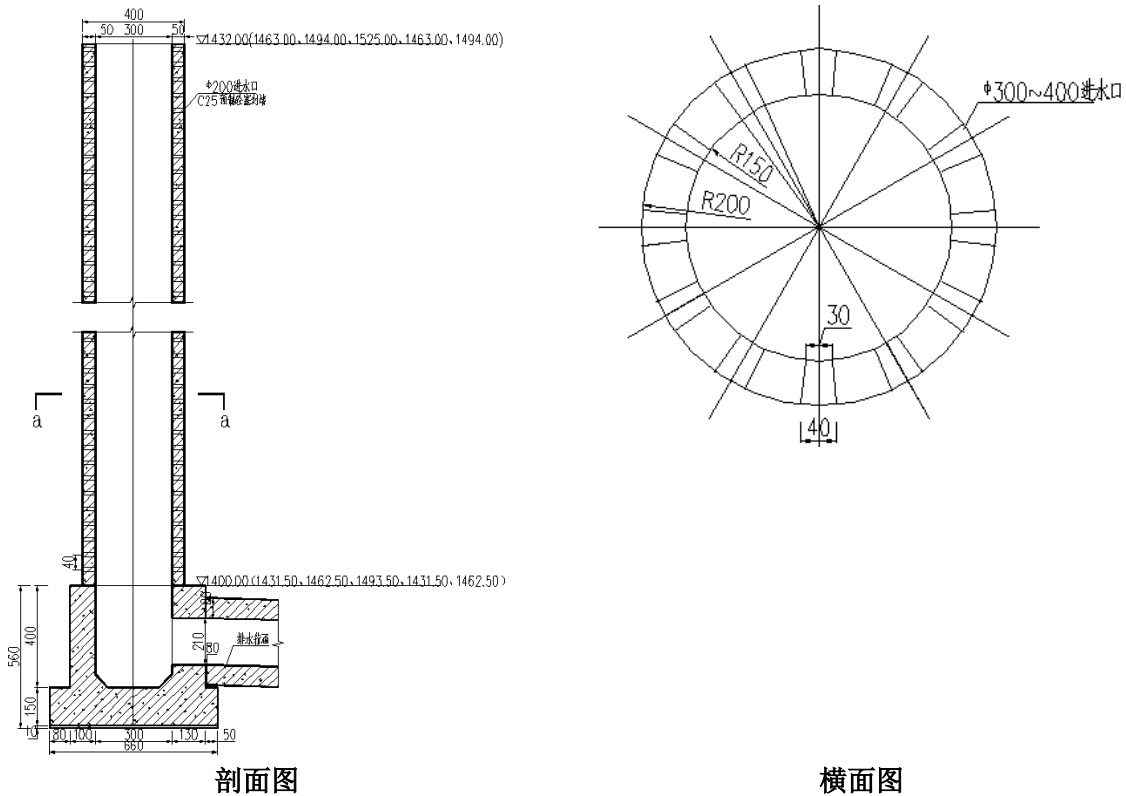
图 2.4.3-1 排水竖井结构断面图
