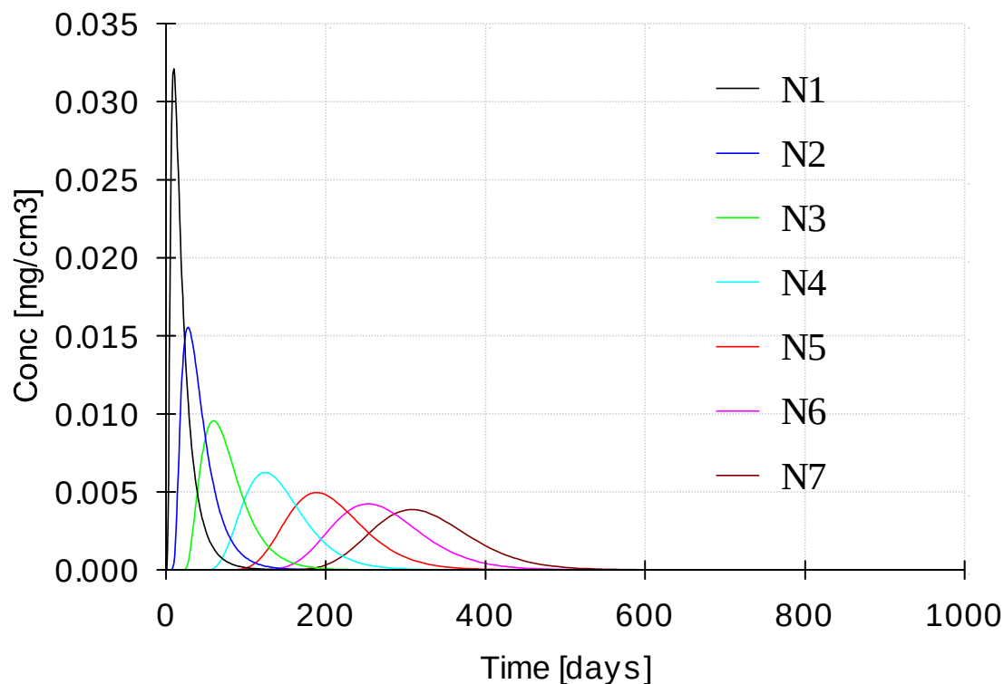
图 5.7-4 当发生废水短时间渗漏 3d 时硫酸盐土壤污染预测图
