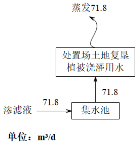
图 3.3-5 本工程封场期水平衡图
