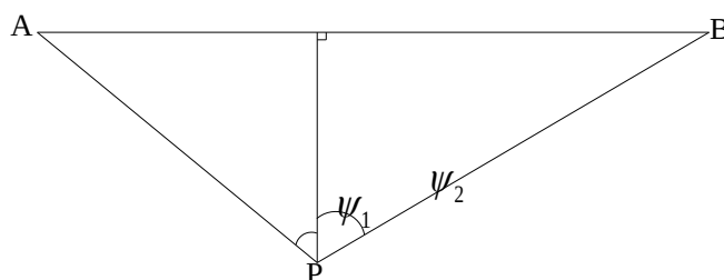
图 5.4.2-1 有限路段的修正函数, A---B 为路段, P 为预测点
