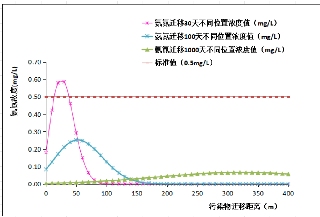
图 5.3.2-14 事故状况下污染物氨氮向南侧迁移不同时间不同位置距离浓度曲线图
