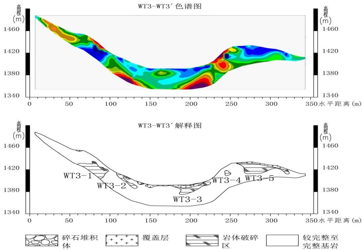
图 4.2.3-5 初期轴线高密度电法测试异常解译图
