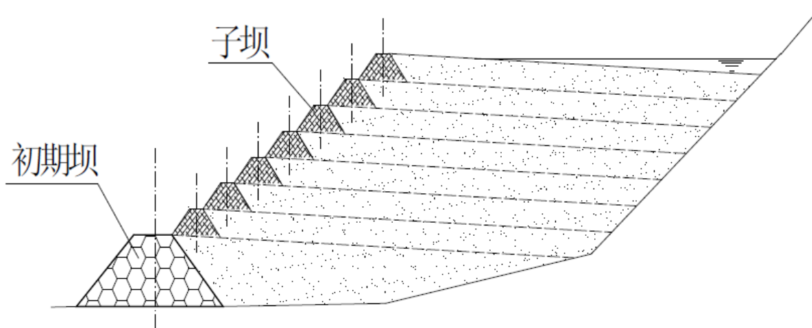
图 2.4-1 上游式堆积坝堆筑示意图
