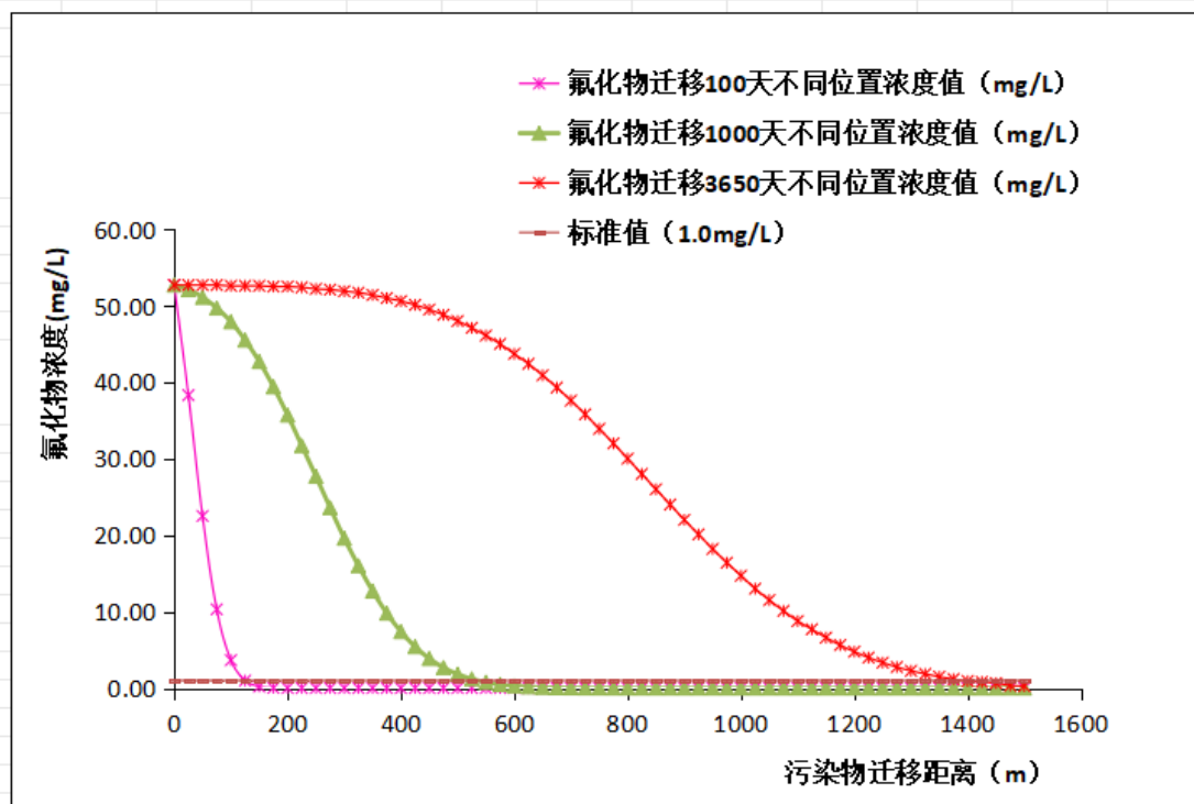
图 5.3.2-7 非正常状况下污染物氟化物向南西侧迁移不同时间不同位置距离浓度曲线图
