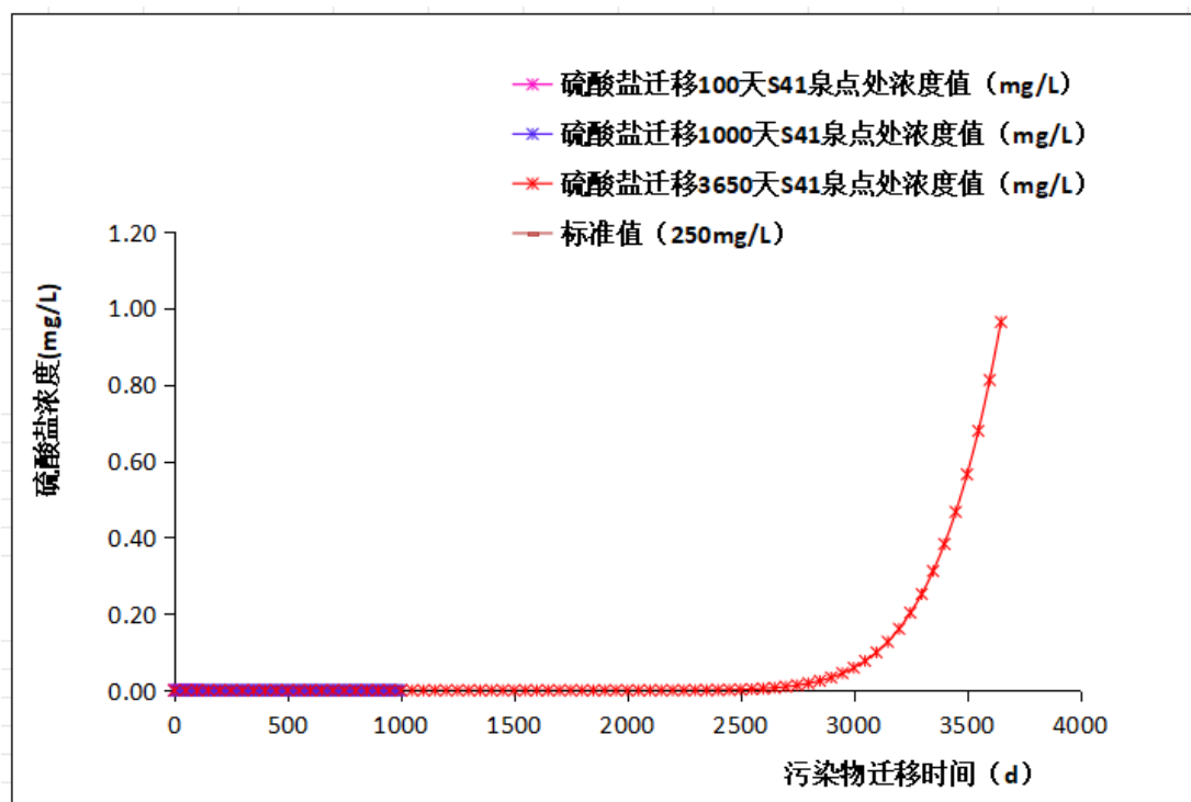
图 5.3.2-12 非正常状况下污染物硫酸盐向南侧 S41 号泉点处迁移不同时间浓度曲线图
