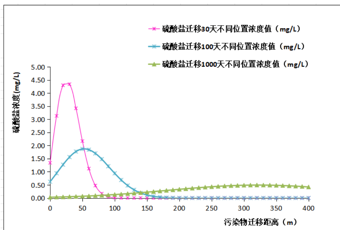
图 5.3.2-6 事故状况下污染物硫酸盐向南侧迁移不同时间不同位置距离浓度曲线图
