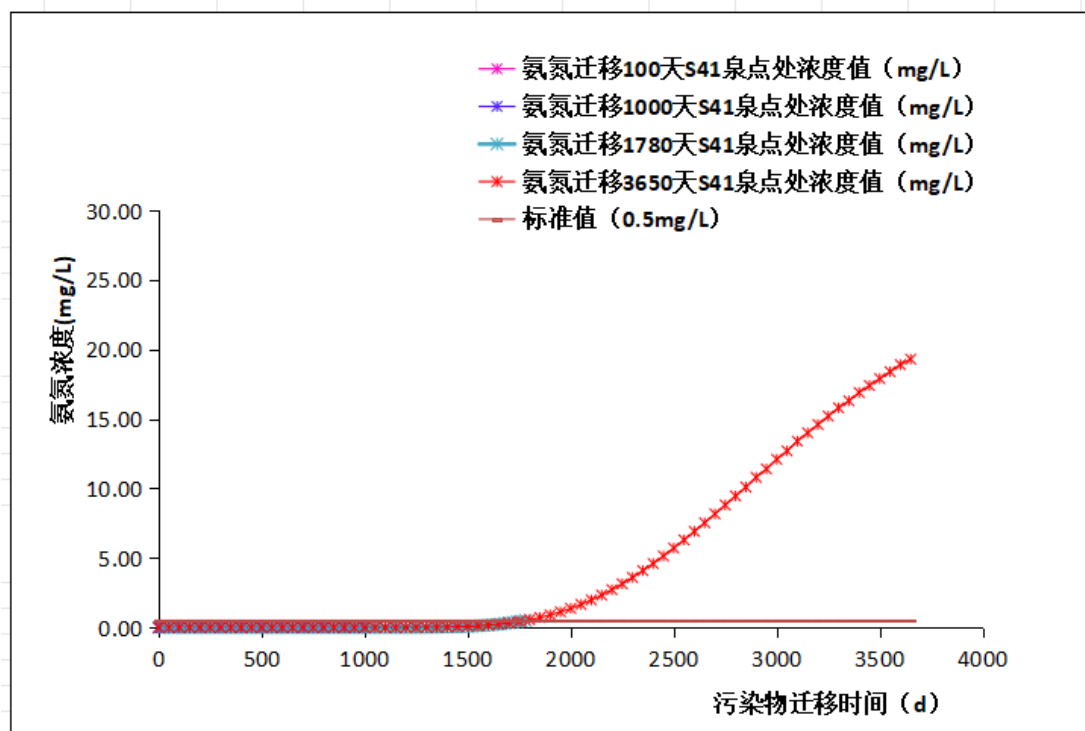
图 5.3.2-4 非正常状况下污染物氨氮向南侧 S41 号泉点处迁移不同时间浓度曲线图
