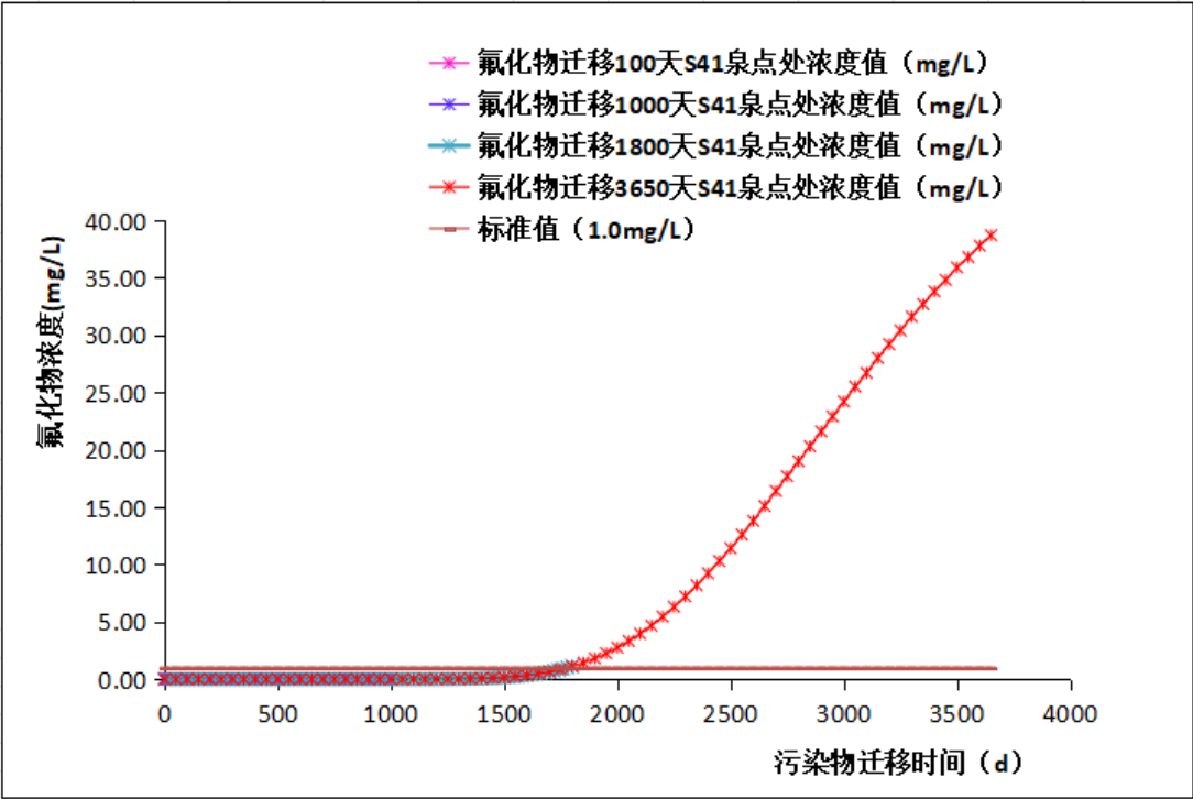
图 5.3.2-2 非正常状况下污染物氟化物向南侧 S41 号泉点处迁移不同时间浓度曲线图
