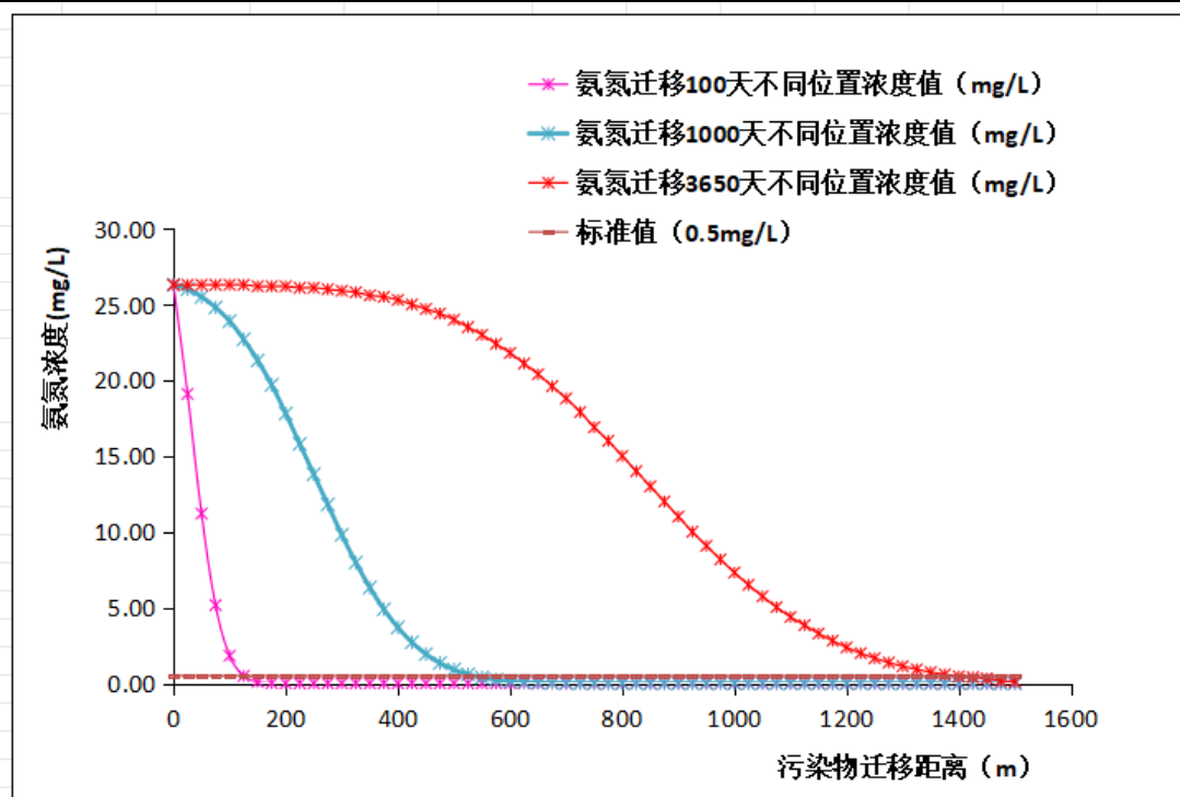
图 5.3.2-9 非正常状况下污染物氨氮向南侧迁移不同时间不同位置距离浓度曲线图
