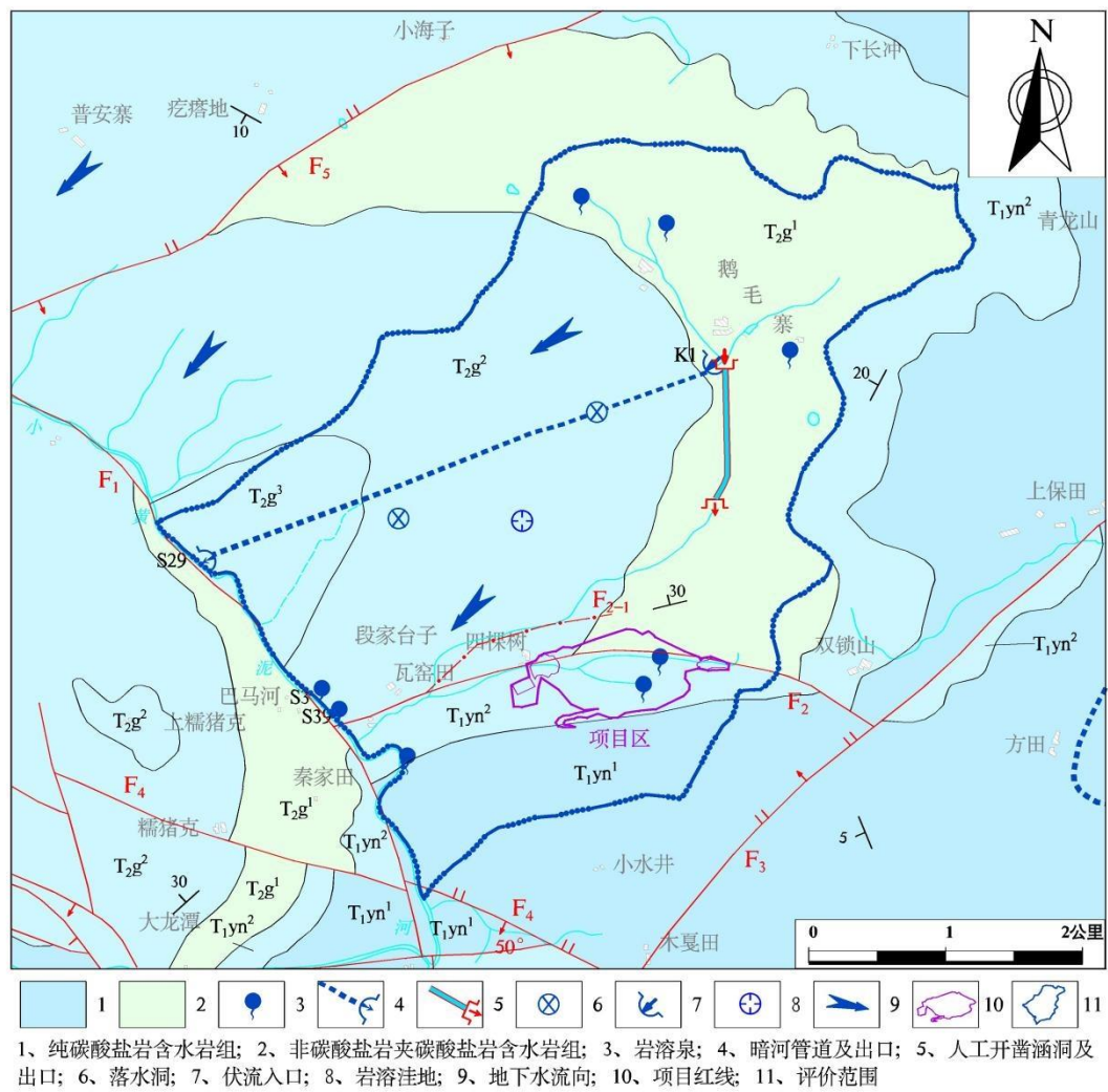
图 4.2.3-3 评价区岩溶个体位置分布图
