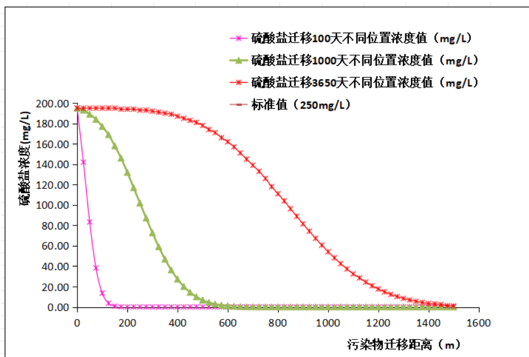
图 5.3.2-11 非正常状况下污染物硫酸盐向南侧迁移不同时间不同位置距离浓度曲线图
