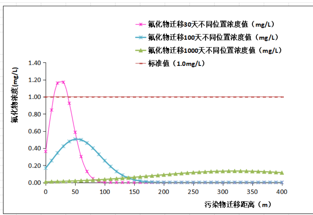
图 5.3.2-13 事故状况下污染物氟化物向南西侧迁移不同时间不同位置距离浓度曲线图
