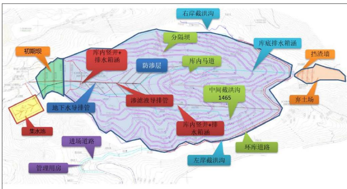
图 2.3-1 处置场总平面布置图
