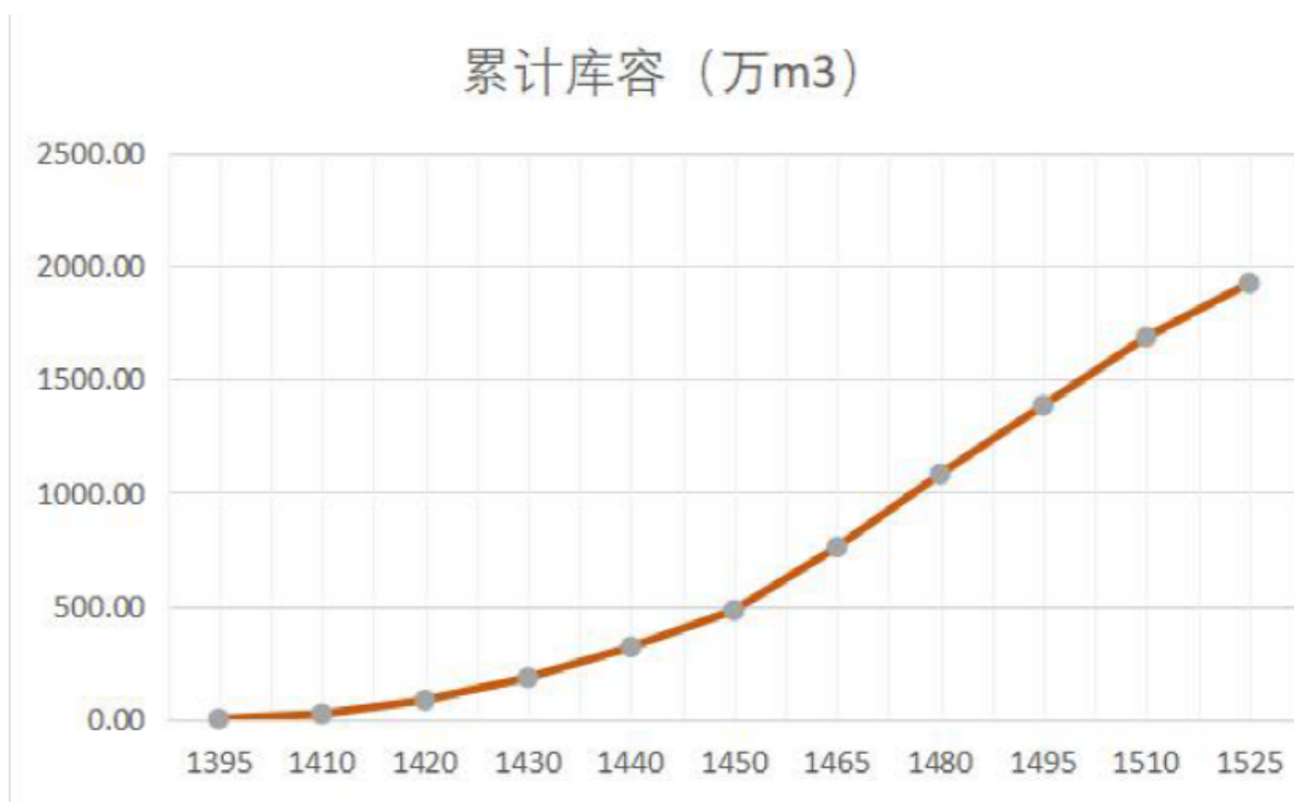
图 2.4.2-1 处置场库容曲线
