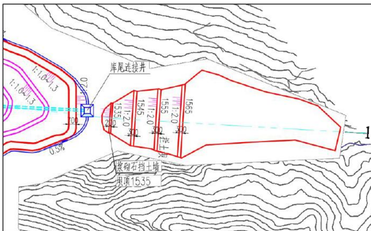
图 2.5.3-1 表土临时堆存场平面布置图
