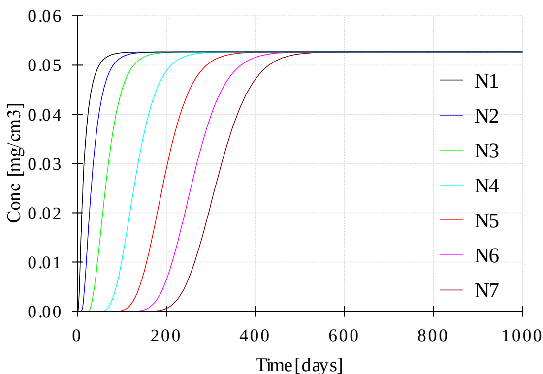
图 5.7-1 当发生废水持续渗漏 1000d 时氟化物土壤污染预测图
