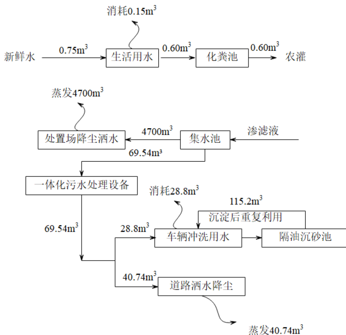
图 3.3-4 本工程营运期水平衡图（超过 3 天但集水池未满）
