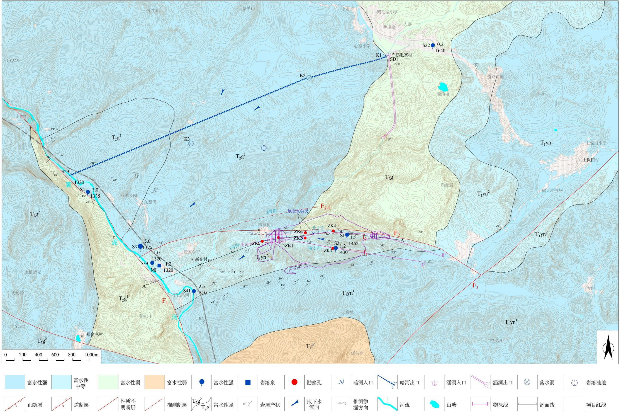
图 4.2.3-7 库区 1:10000 水文地质图
