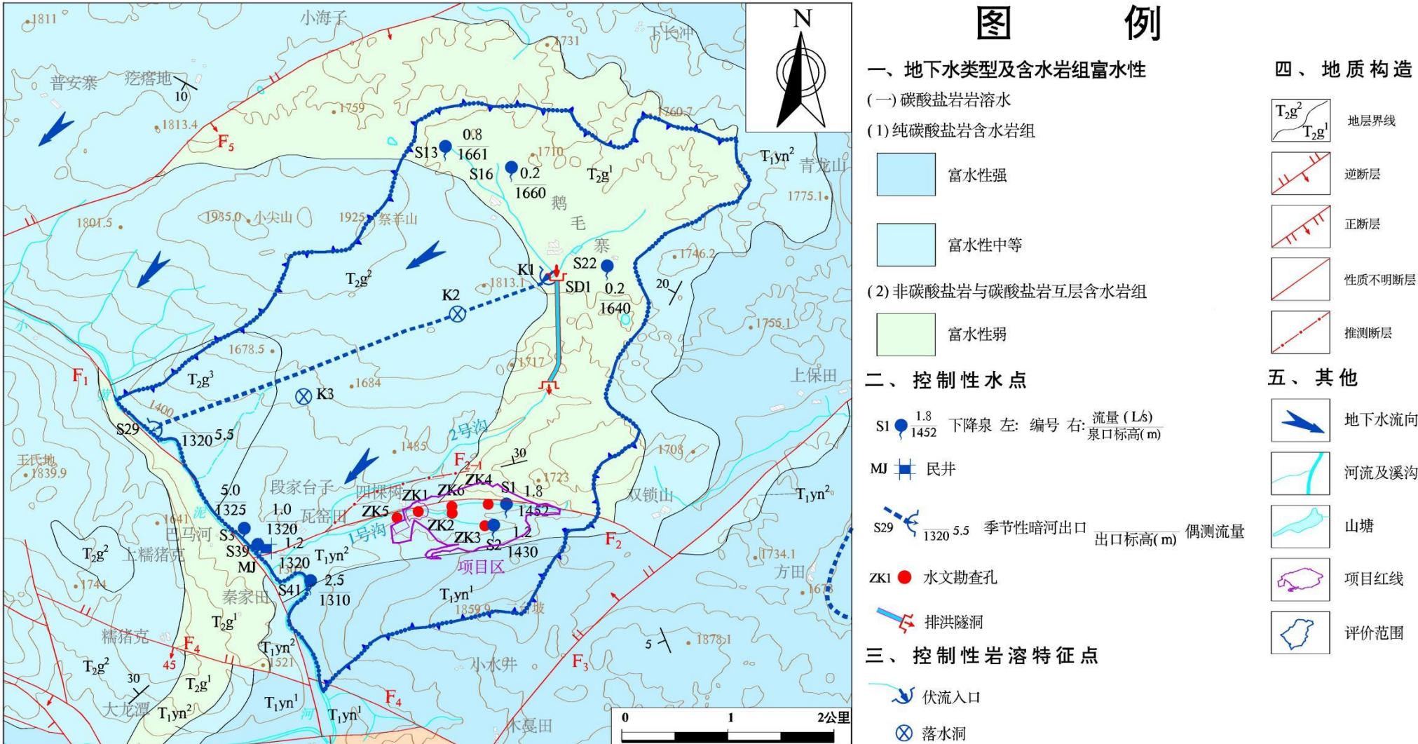
图 4.2.3-6 调查评价区 1:5 万水文地质图
