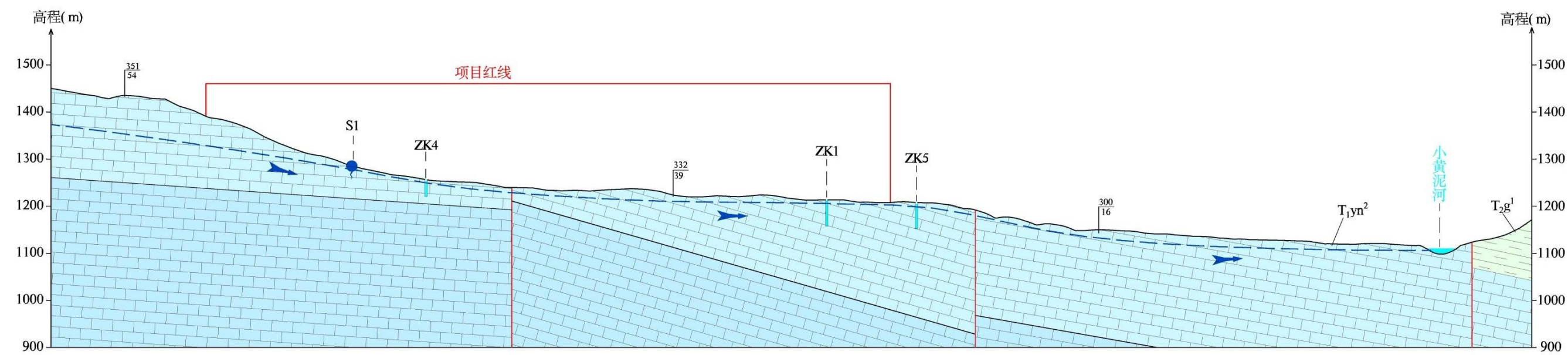
图 4.2.3-8 水文地质剖面示意图
