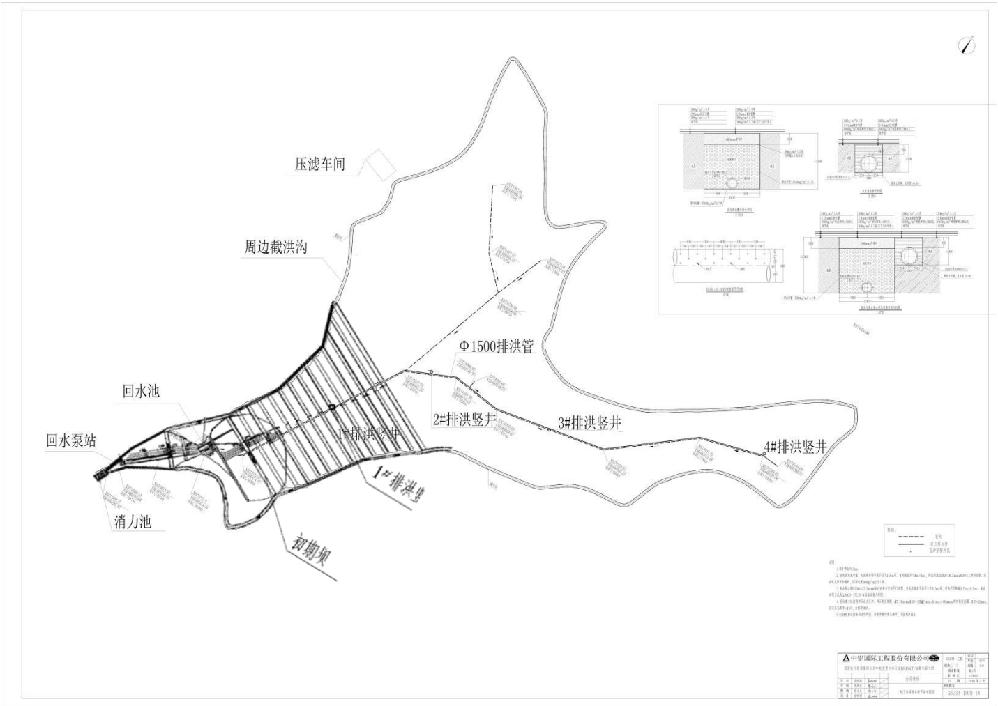
图 2.2-1 现有堆场总平面布置图
