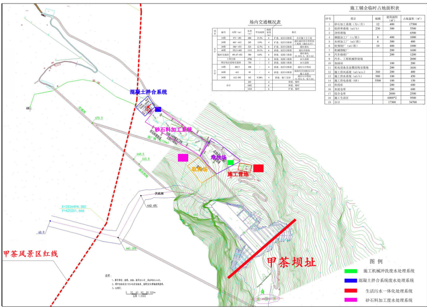
图 2.2-1 原环评阶段施工布置图
