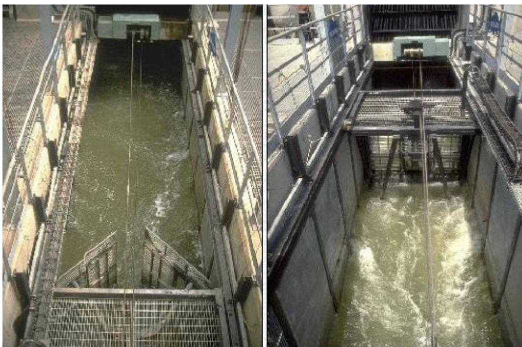
图 6.2-4 集鱼通道实例图
