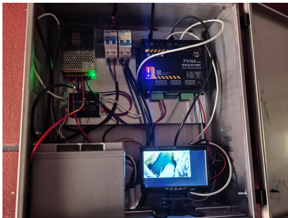
图 6.2-1 生态流量在线监测系统
