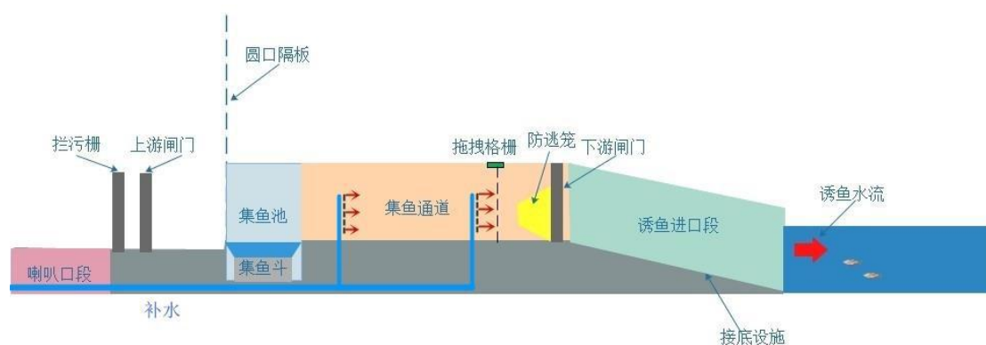
图 6.2-3 鱼系统结构组成示意图（侧视图）
