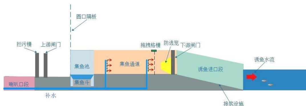
图 6.2-6 补水系统示意图
