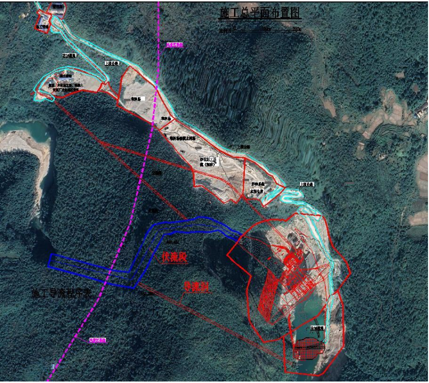
图 2.2-2 实际施工布置图
