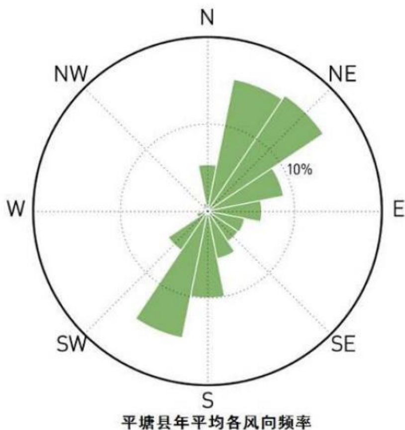
图 4.1-1 项目涉及区风玫瑰图
