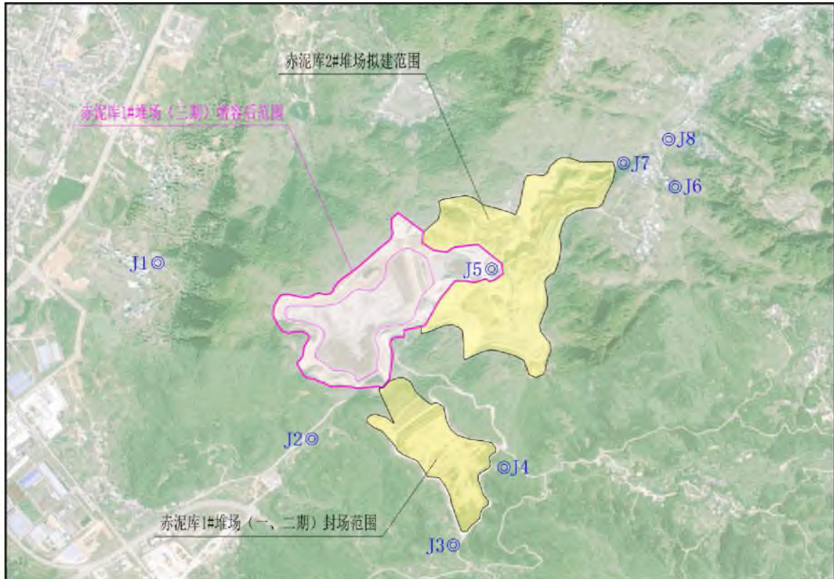
赤泥堆场周边地下水监测井布置示意图
