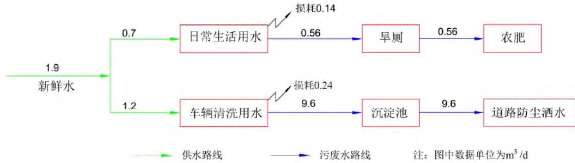
办公区水量平衡图
