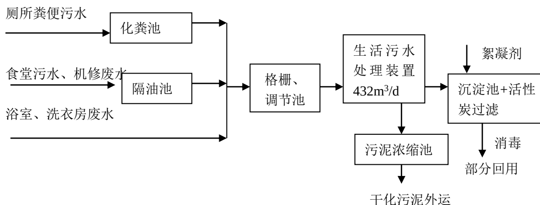
图 5.3-3 生产、生活污水处理工艺流程图
