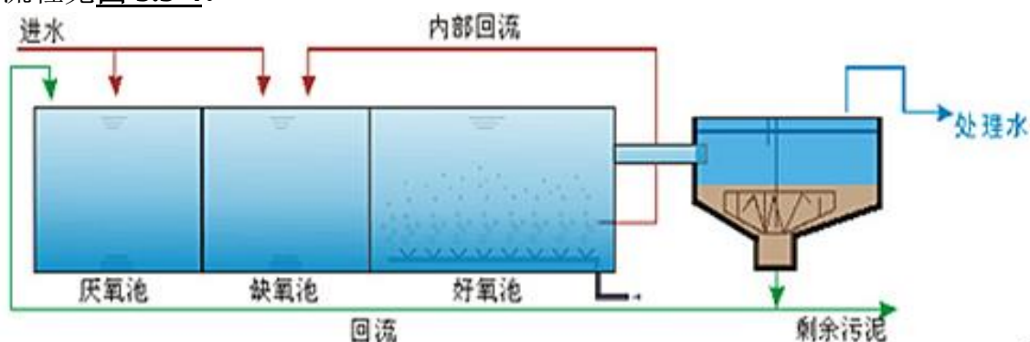
图 5.3-4 A^2/O 工艺流程图
