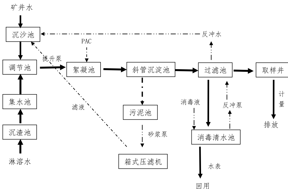
图 5.3-1 矿井水处理工艺流程
