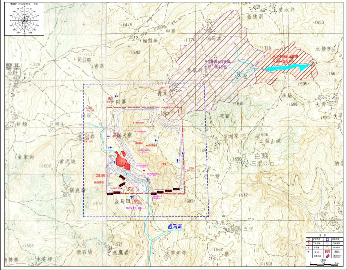
附图4.3-2 全井田沉陷等值线图
