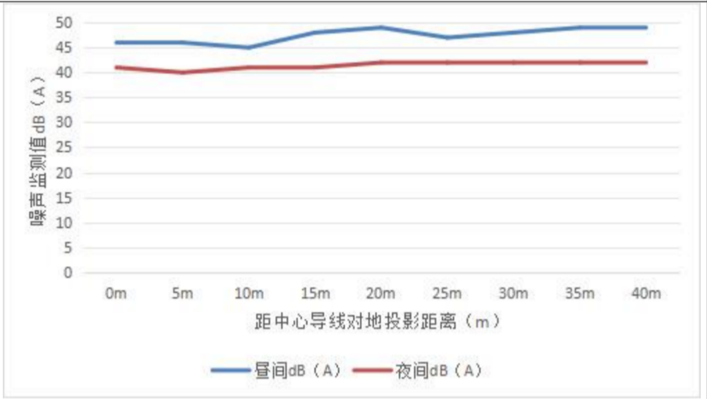
图 4-5 广州市 220kV 森从甲线噪声监测断面衰减趋势示意图
