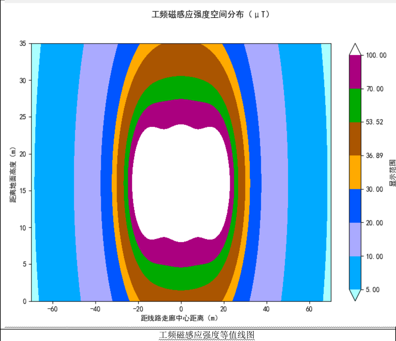
图 6-2 本项目改造线路工频磁场分布图
