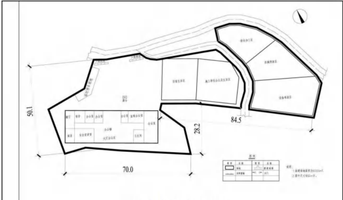
图 2-1 施工总平面布置图
