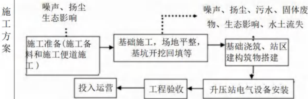
图 2-2 施工工艺流程及产污节图
