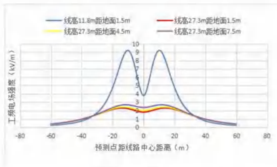
图 5.2-1 工频电场强度计算结果分布曲线图
