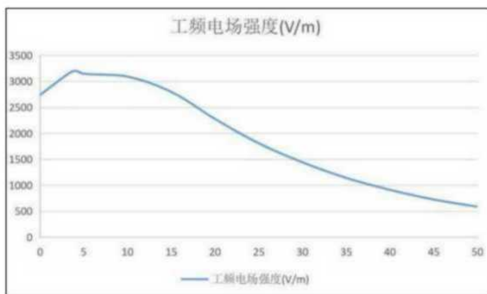
图 5.2-3 类比单回输电线路工频电场强度监测衰减断面趋势图
