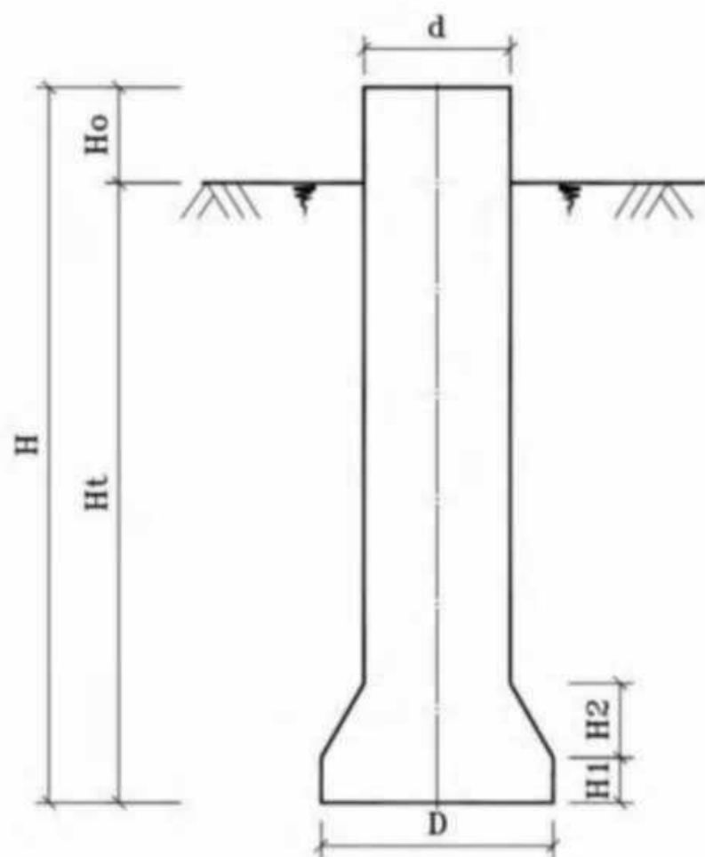
附图 5.1-1 生态环境保护措施设计图（挖孔桩基础）
