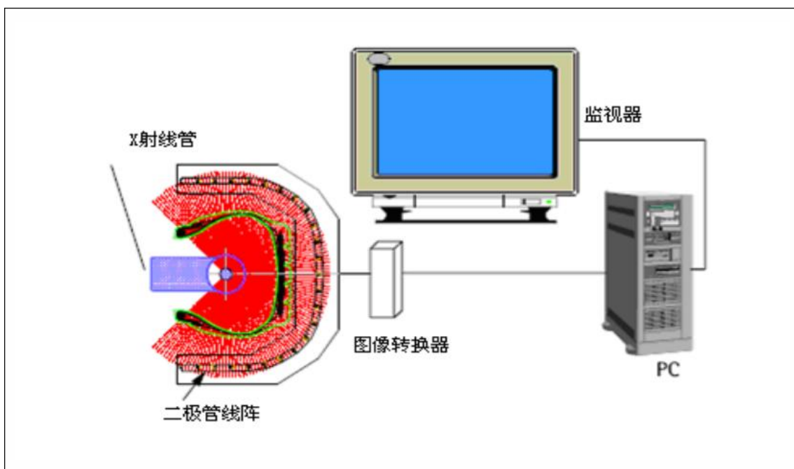
图9-3 X射线成像系统原理图
