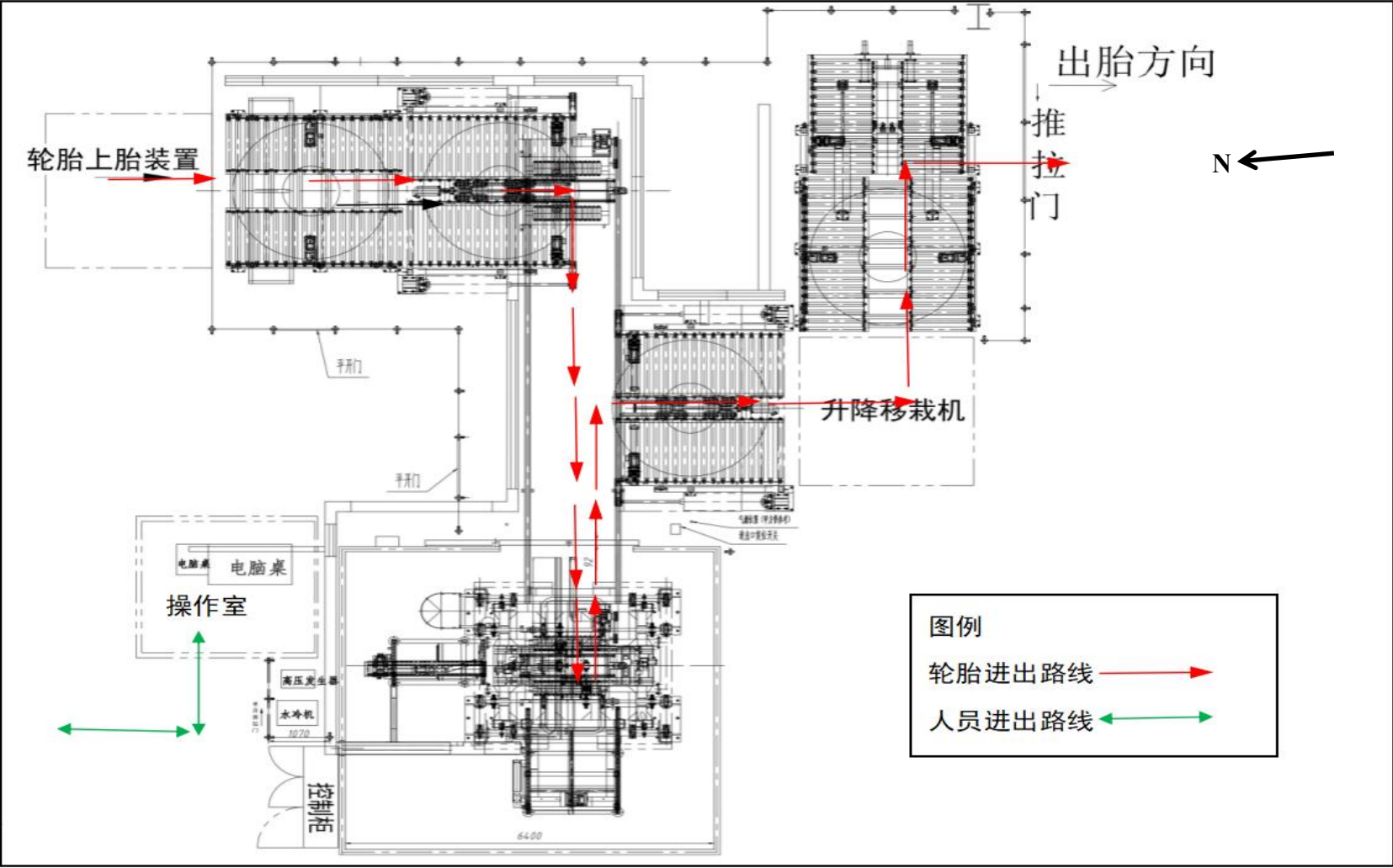
附图 5 本项目人流物流示意图
