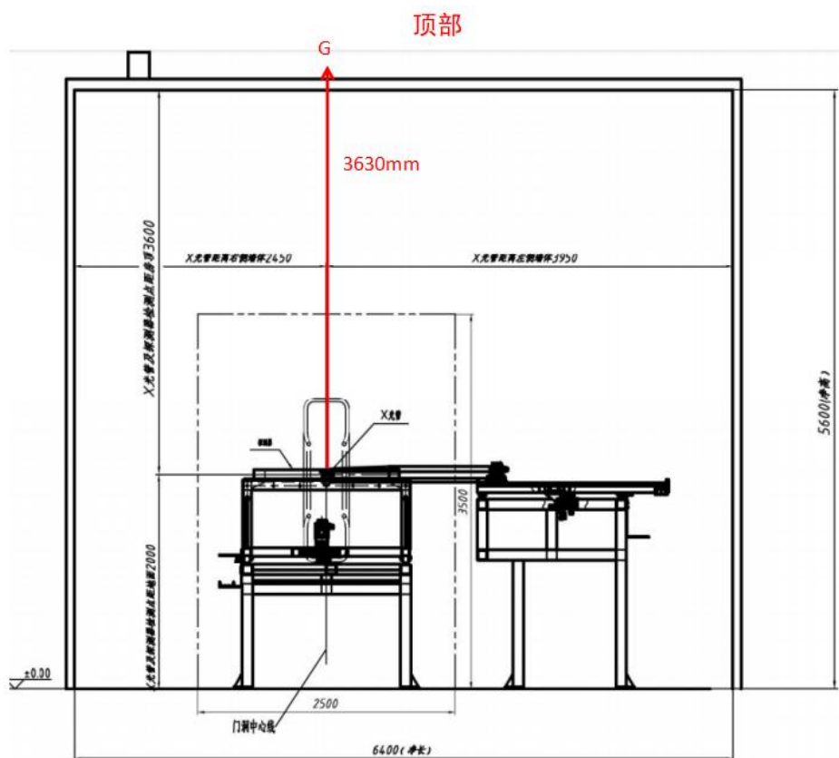
图 11-3 铅房顶部关注点位剖面分布示意图
