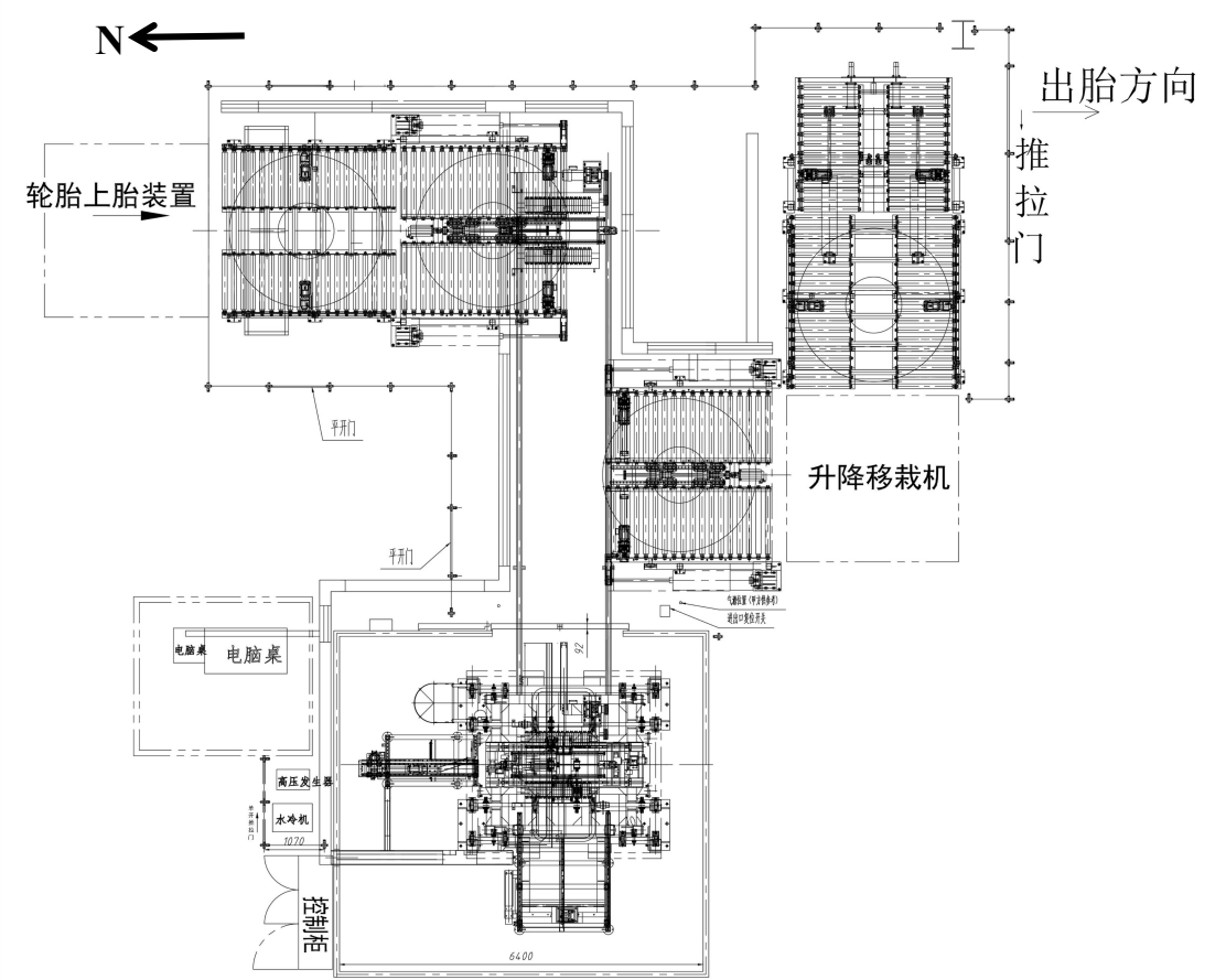
图9-1 设备总体结构图
