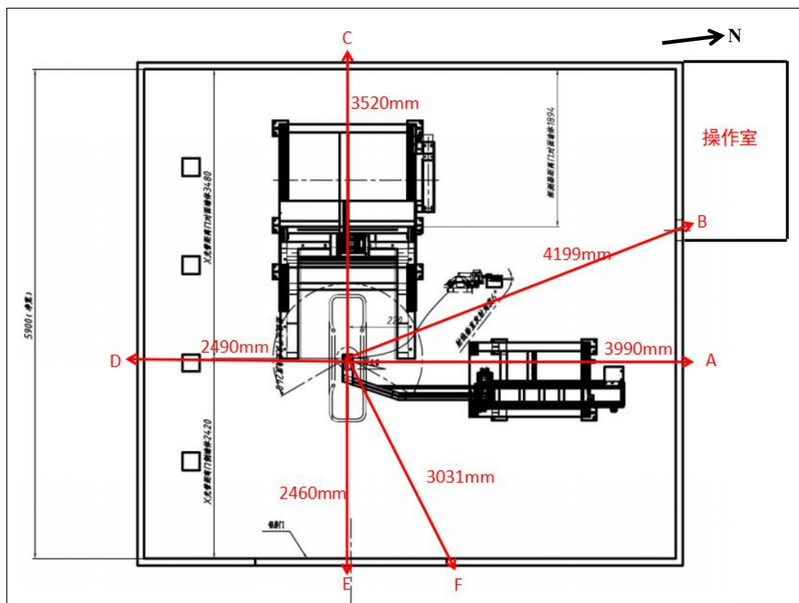
图 11-2 铅房周围关注点位平面分布示意图
