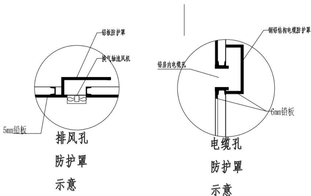
图 10-4 排风孔防护罩及电缆孔防护罩屏蔽设计图
