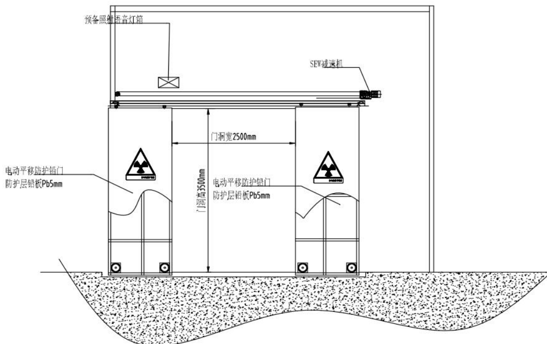
图 10-3 铅房门屏蔽设计图
