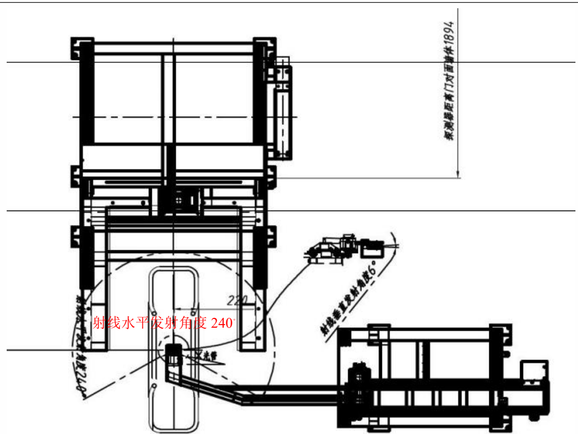
图9-2 设备结构示意图
