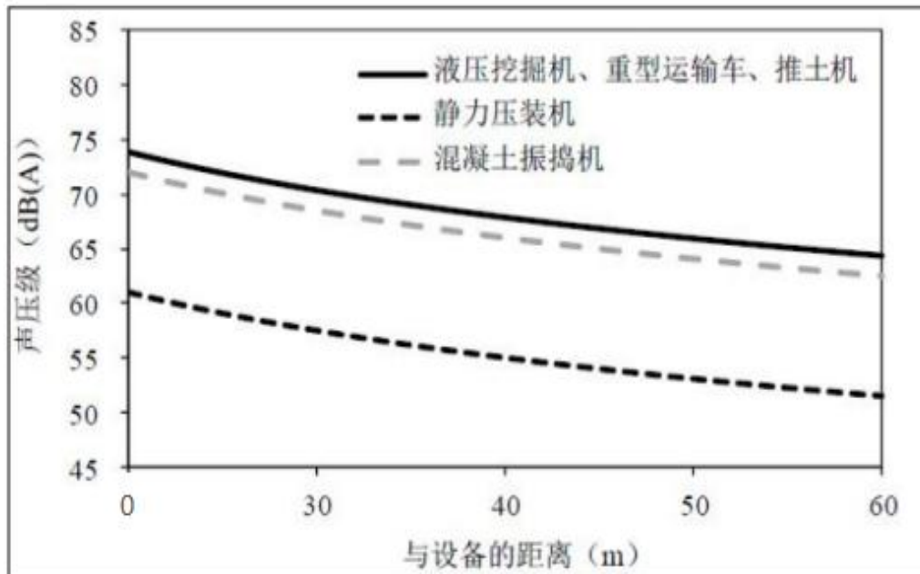
图 4.1 施工设备声环境影响预测结果
