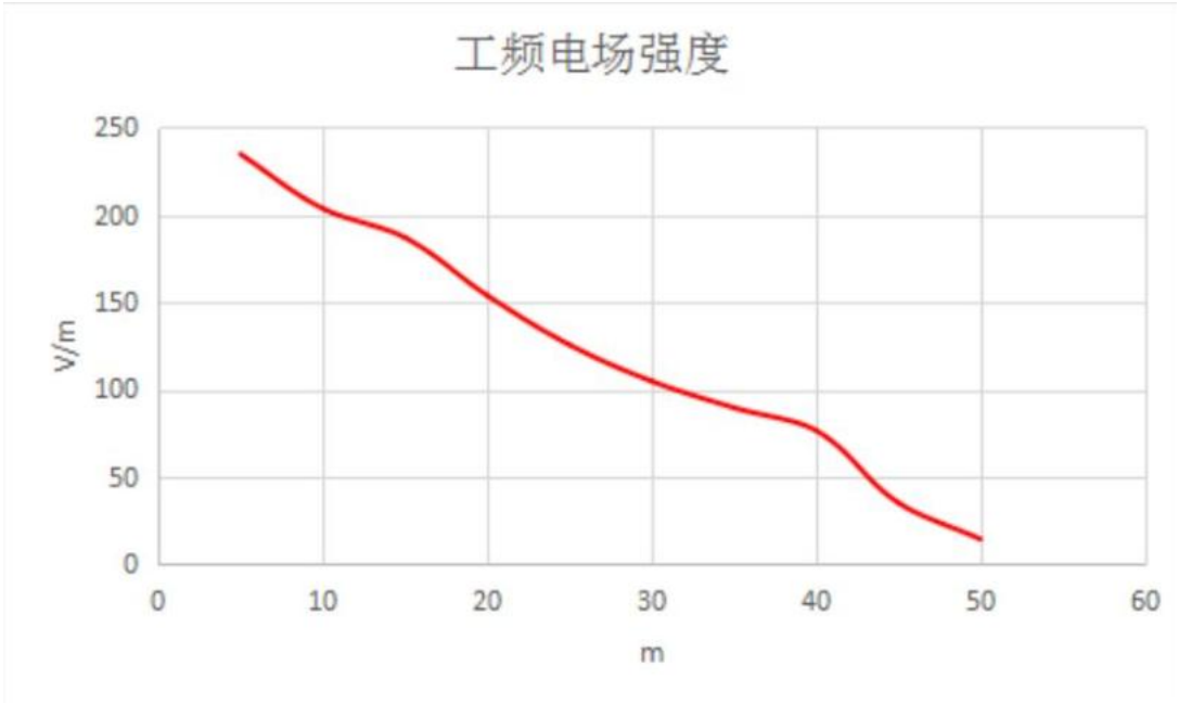
图 4.2-3 类比变电站工频电场强度变化趋势图
