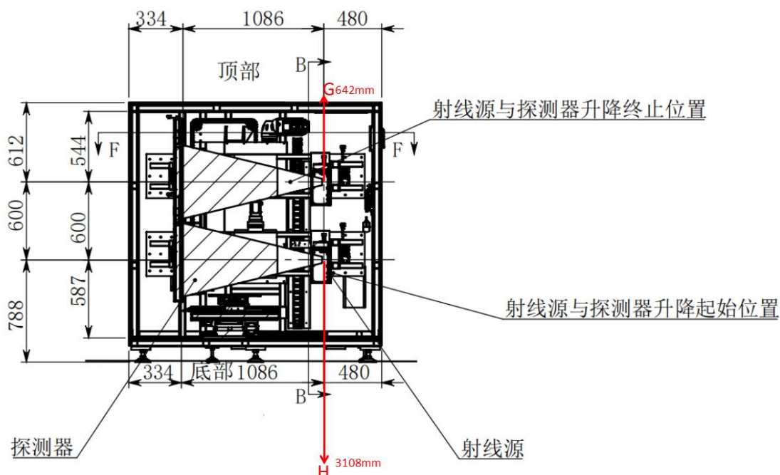
图 11-1 射线源分布及关注点位示意图（剖面图）
