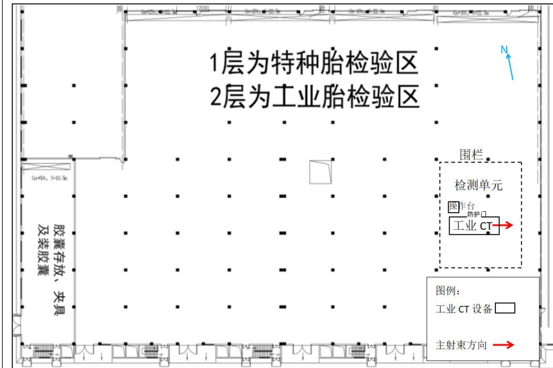
图 11-5 主射束朝东侧照射时工业 CT 安装摆放示意图
