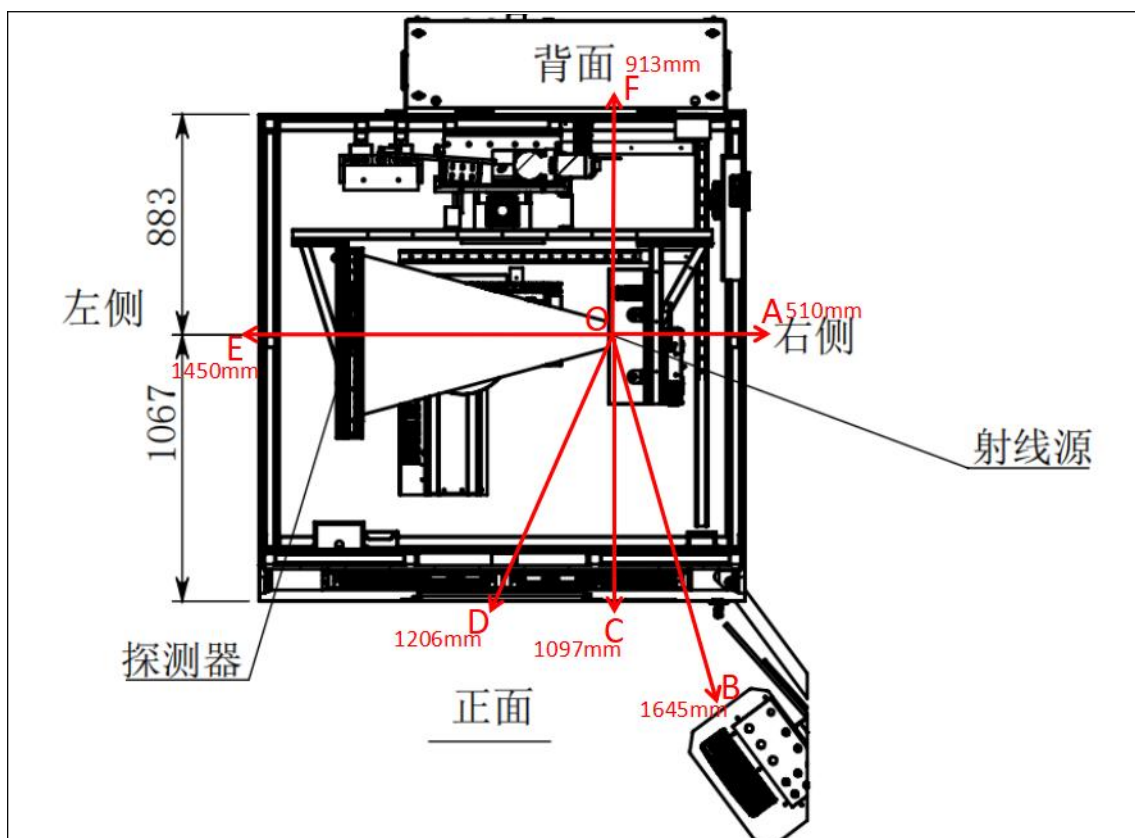
图 11-2 射线源分布及关注点位示意图（俯视图）
