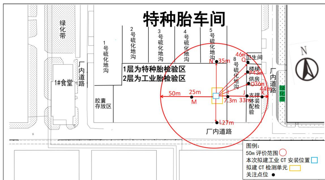
图 11-3 50m 范围内关注点位示意图
