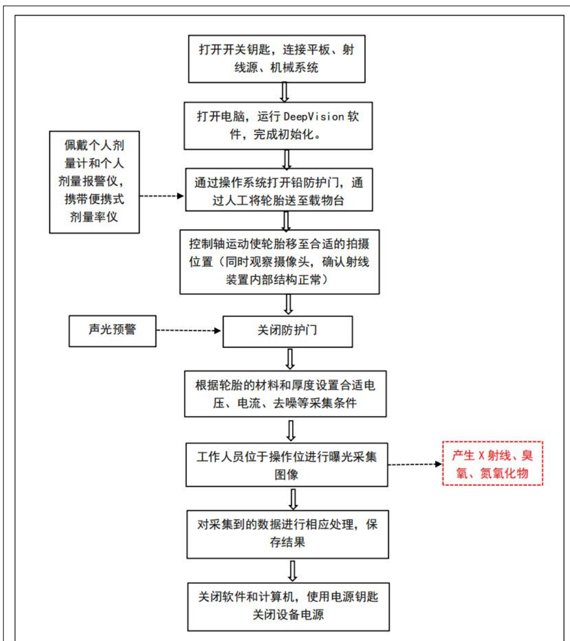
图 9-4 本项目工艺流程及产污环节示意图
