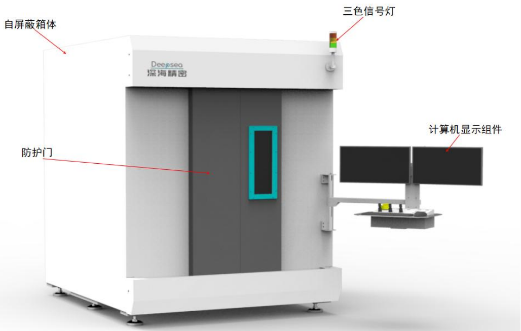
图 9-1 工业 CT 外观图
