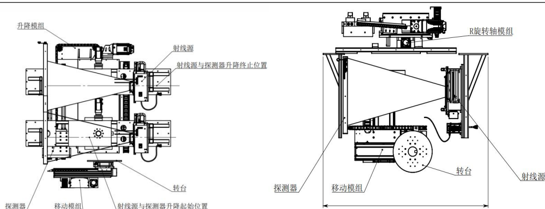
图 9-2 工业 CT 内部结构示意图
