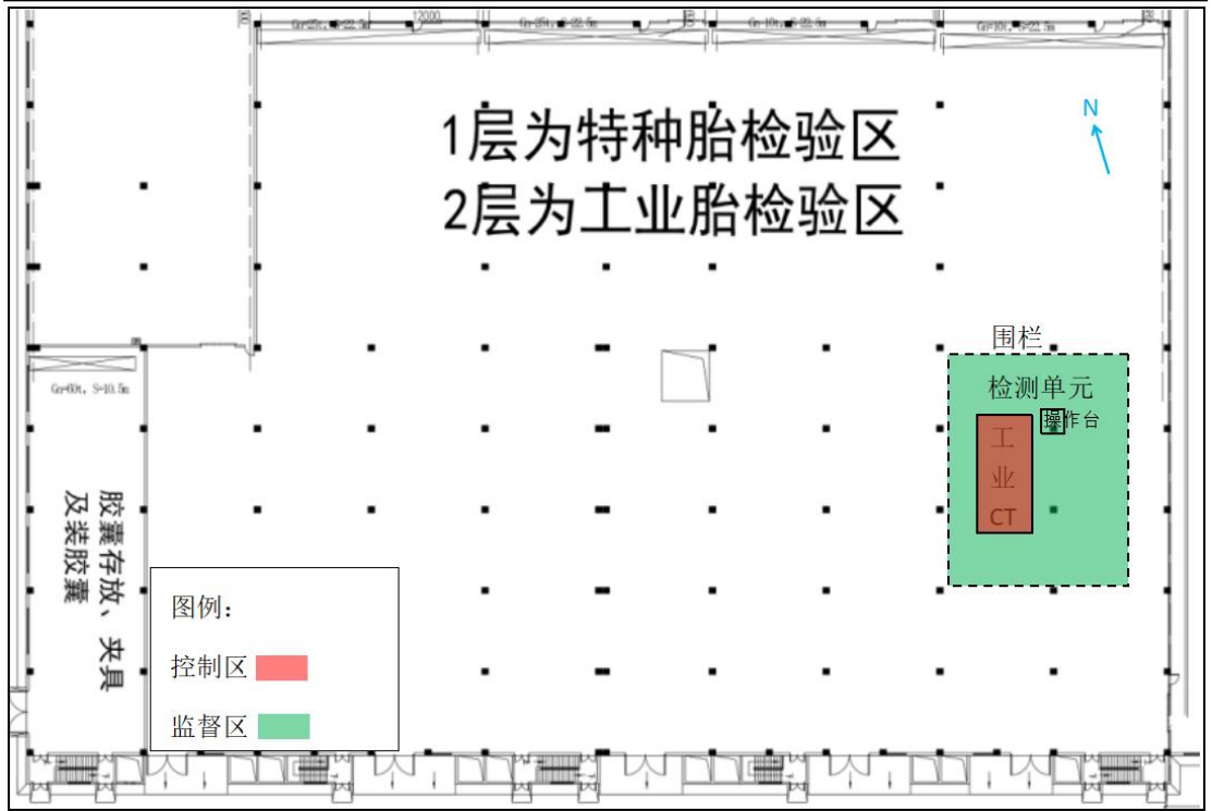
图 10-1 本项目辐射工作场所的分区示意图
