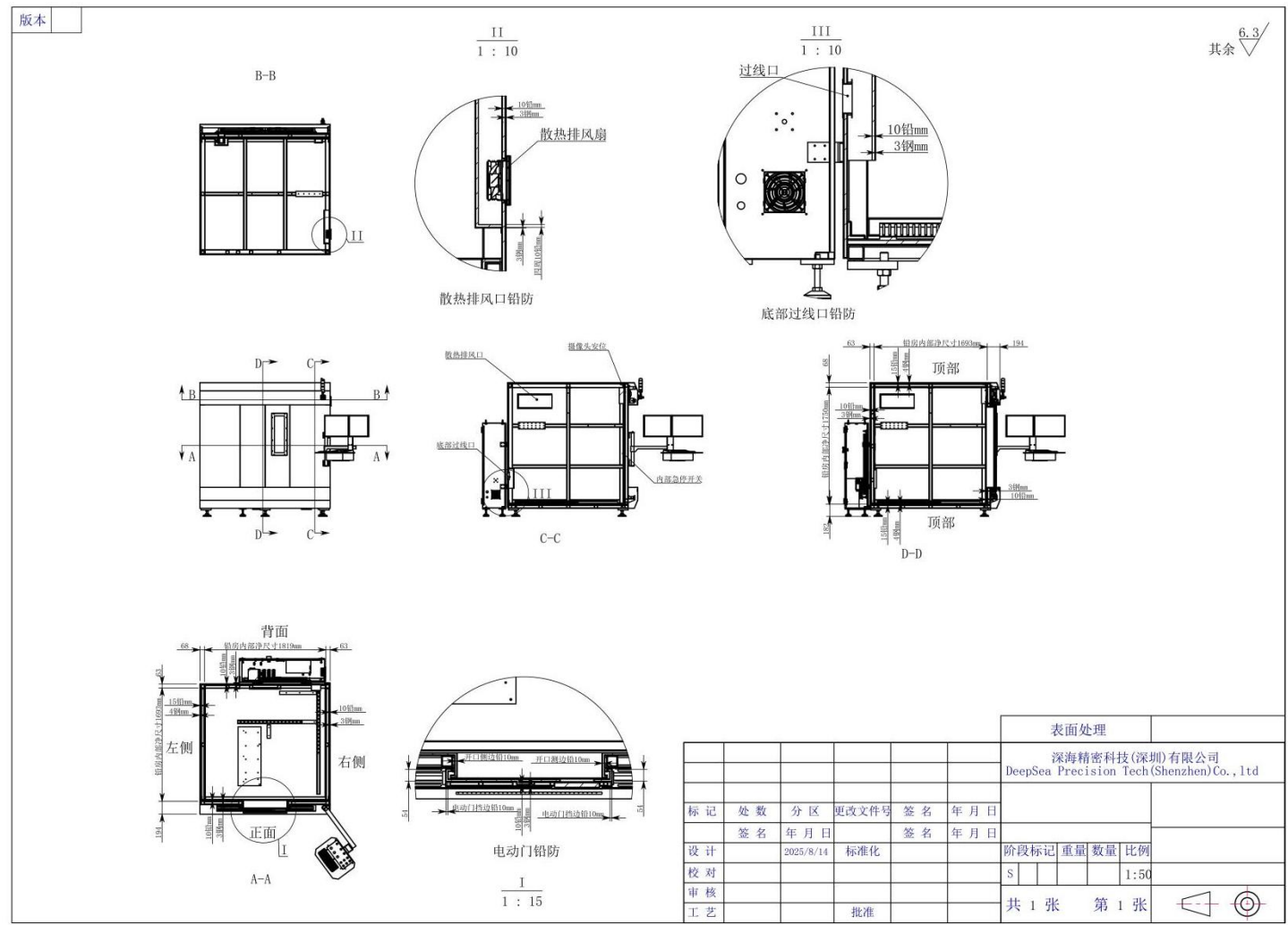
附图 4 本项目屏蔽设计示意图
