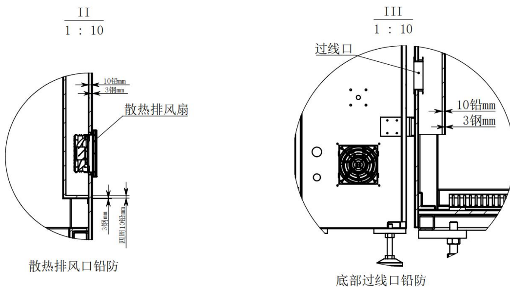
图 10-4 铅房排风口及过线口屏蔽设计示意图
