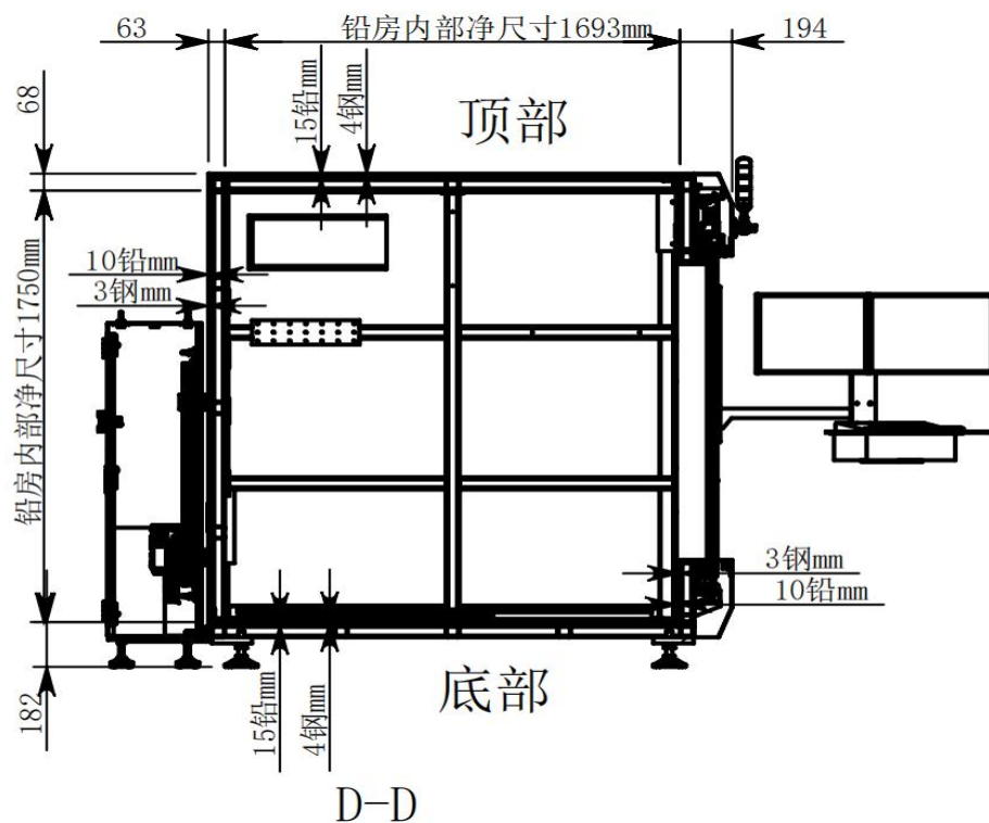
图 10-3 铅房剖面屏蔽设计示意图
