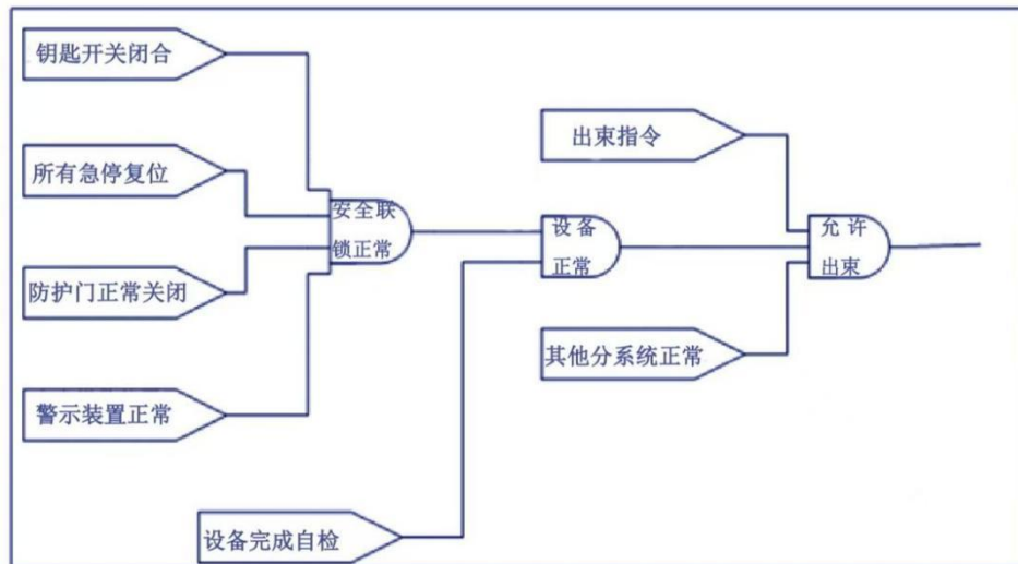
图 10-6 安全联锁逻辑图
