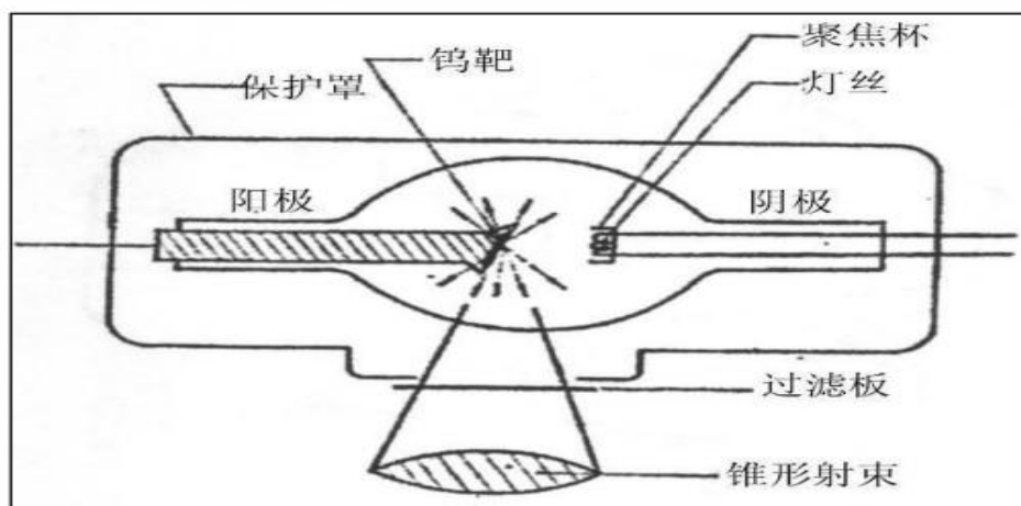
图 9-3 X 射线管示意图
