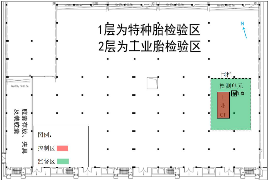
附图 5 本项目工作场所分区示意图
