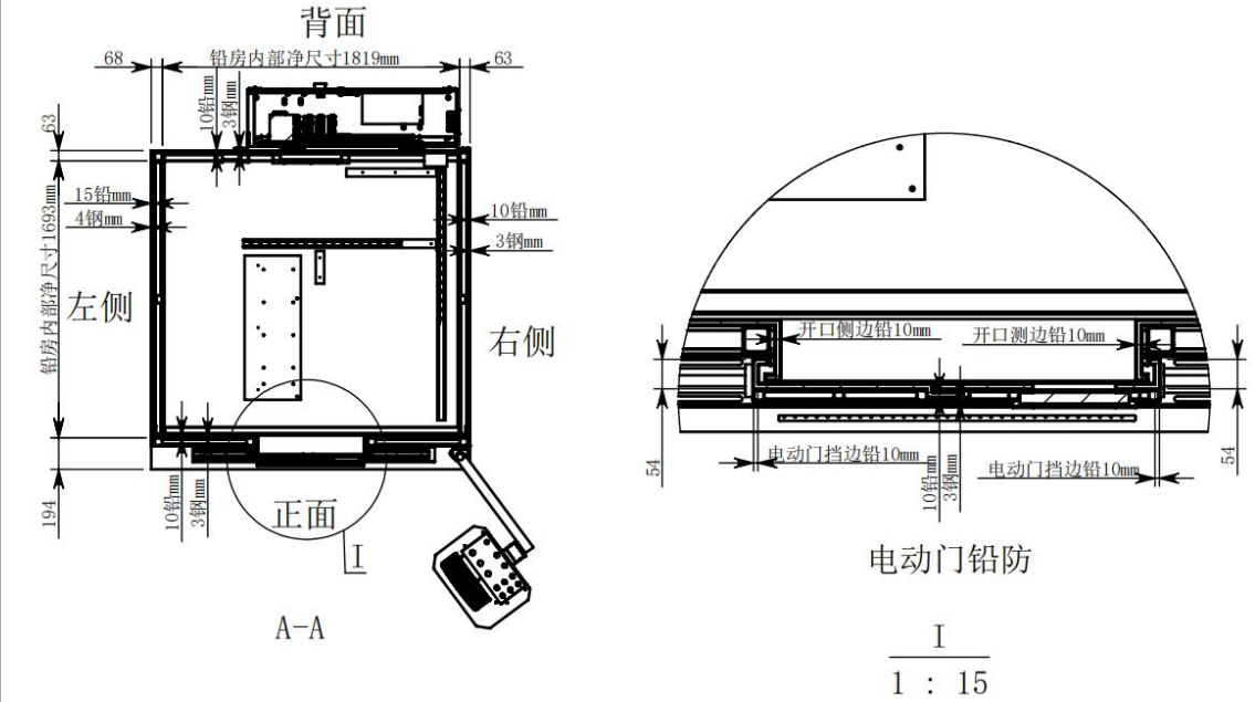
图 10-2 铅房平面屏蔽设计示意图
