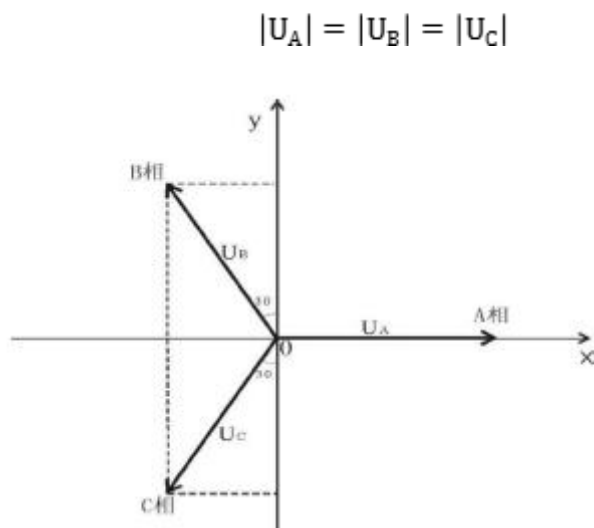
图 C-1 对地电压计算图
