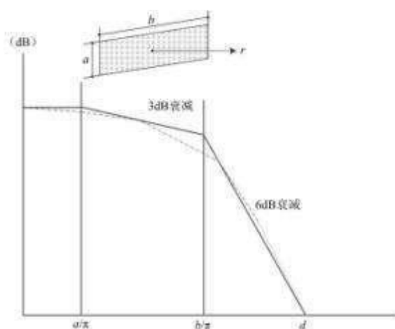
图 6-38 长方形面声源中心轴线上的衰减特性
