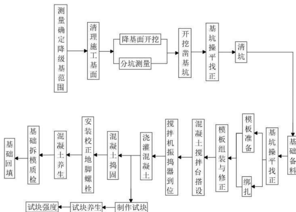
图 3-3 输电线路塔基施工流程图
