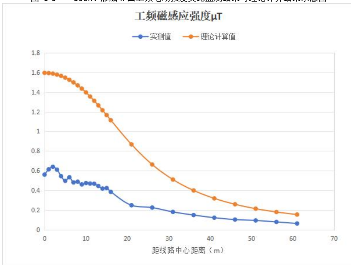
图 6-7 500kV 雁船 II 回工频磁感应强度类比监测结果与理论计算结果示意图
