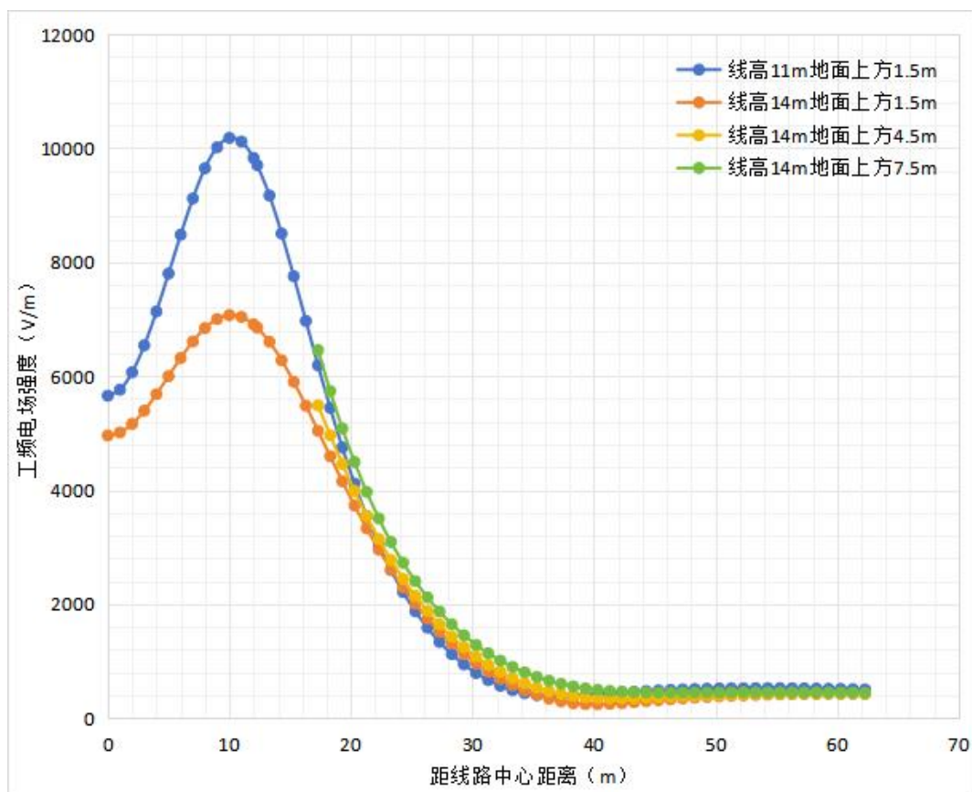
图 6-28 新建 500kV 同塔双回线路工频电场强度分布图
