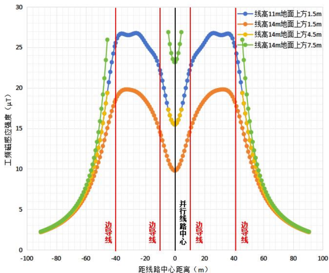
图 6-17 新建 500kV 单回并行线路工频磁感应强度分布图
