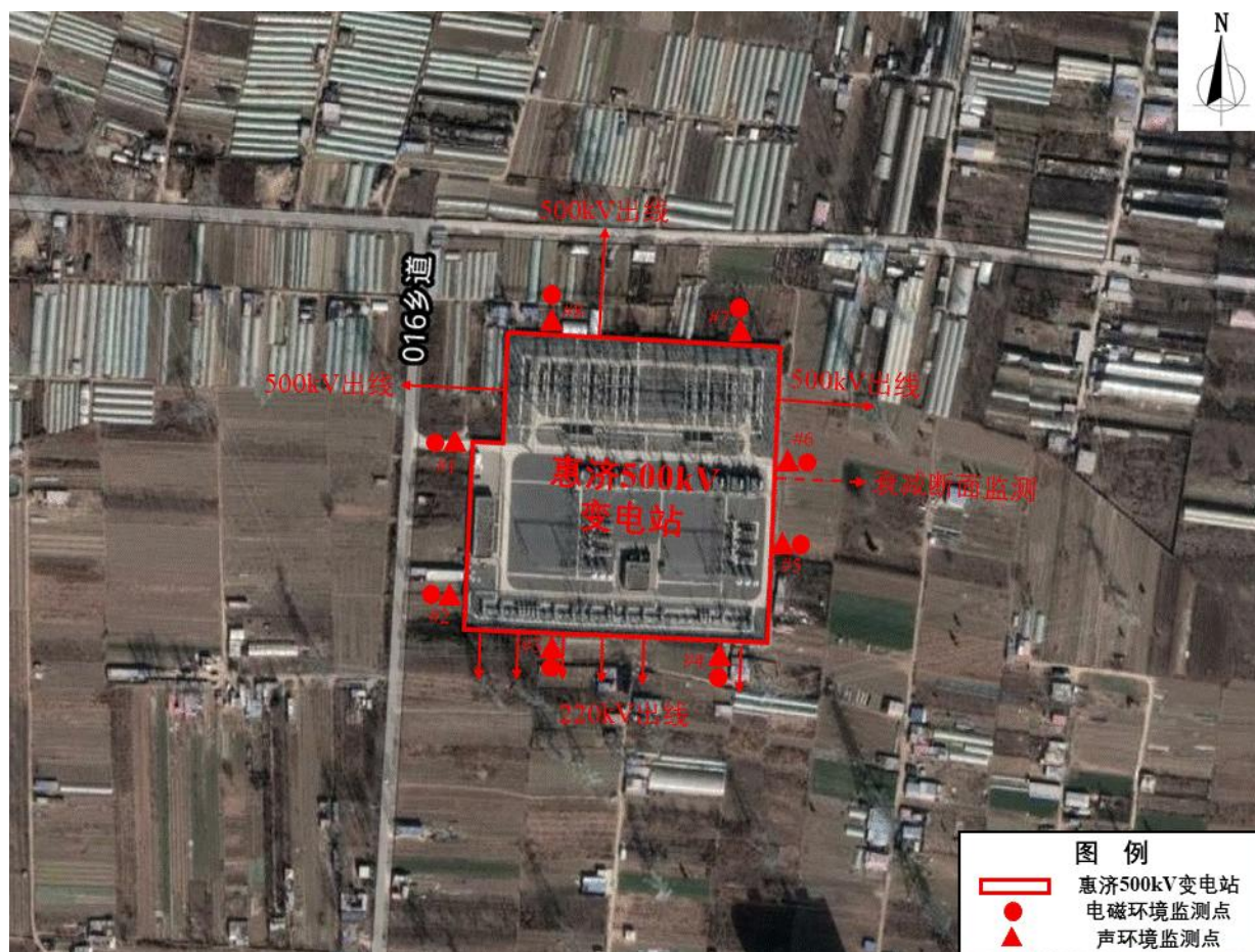
图 6-1 惠济 500kV 变电站厂界电磁环境监测点位示意图
