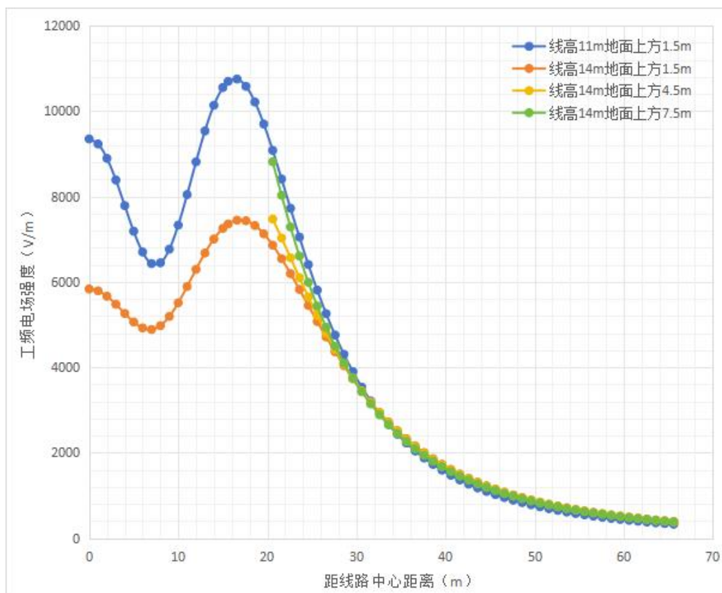
图 6-10 新建 500kV 单回线路工频电场强度分布图
