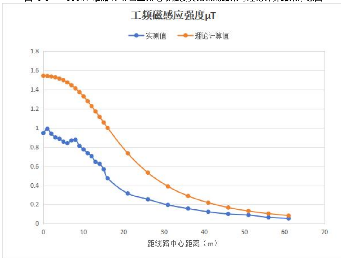
图 6-9 500kV 雁船 I、II 回工频磁感应强度类比监测结果与理论计算结果示意图
