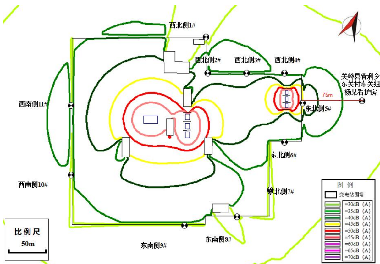
图 6-42 关岭 500kV 变电站本期噪声贡献值等值线分布图（预测点高 1.2m）
