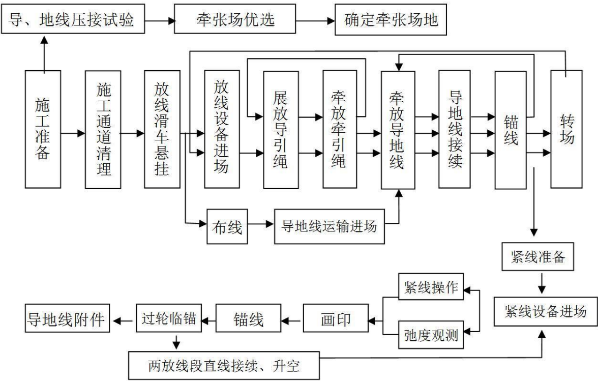
图 3-5 输电线路架线施工流程图
