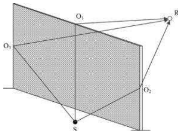
图 6-40 在有限长声屏障上不同的传播路径
