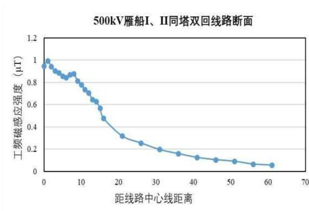
图 6-5 500kV 雁船 I、II 同塔双回线路断面工频电场强度、磁感应强度变化趋势图
