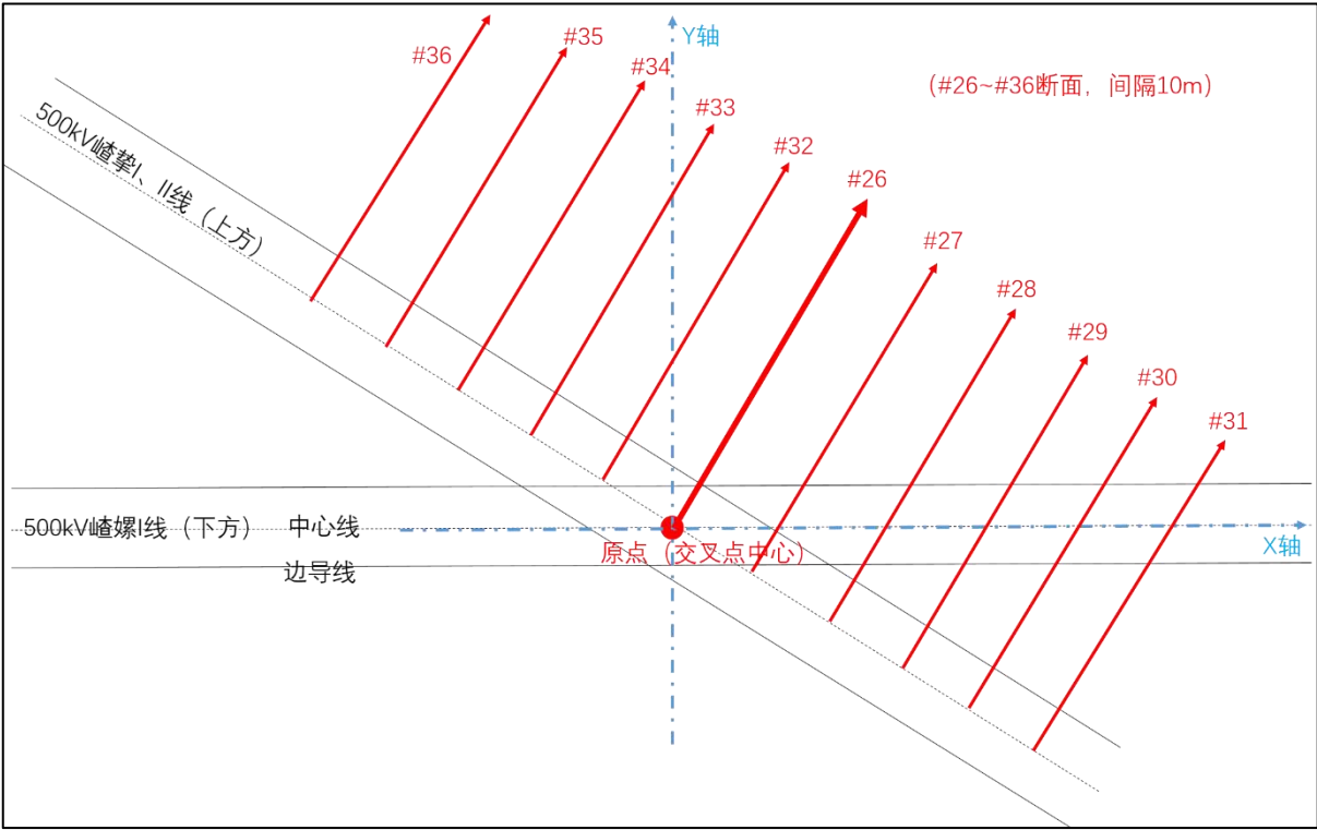
图 6-35 500kV 嵇摯 I、II 线断面监测布设示意图
