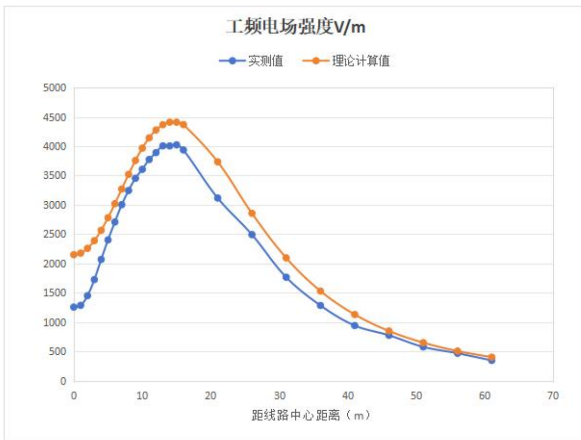
图 6-6 500kV 雁船 II 回工频电场强度类比监测结果与理论计算结果示意图
