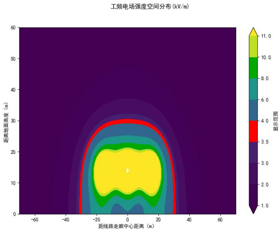
图 6-14 500kV 单回线路居民区工频电场等值线预测图
