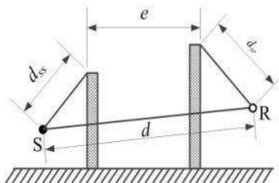
图 6-41 利用建筑物、土堤作为厚屏障
