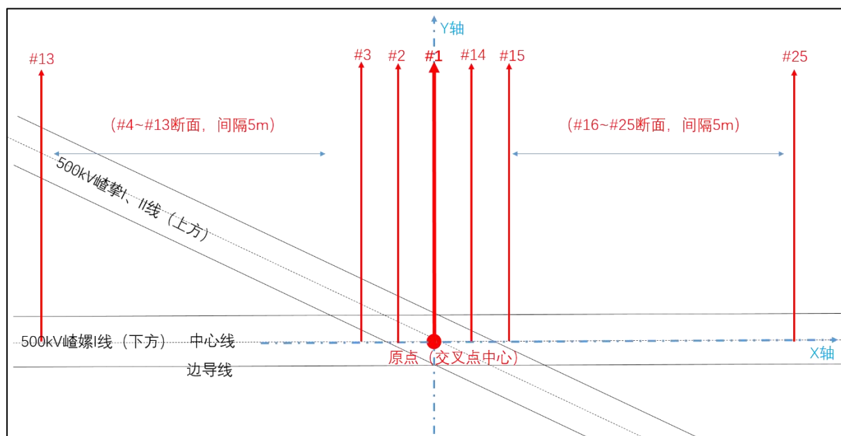
图 6-34 500kV 嵯螺 I 线断面监测布设示意图
