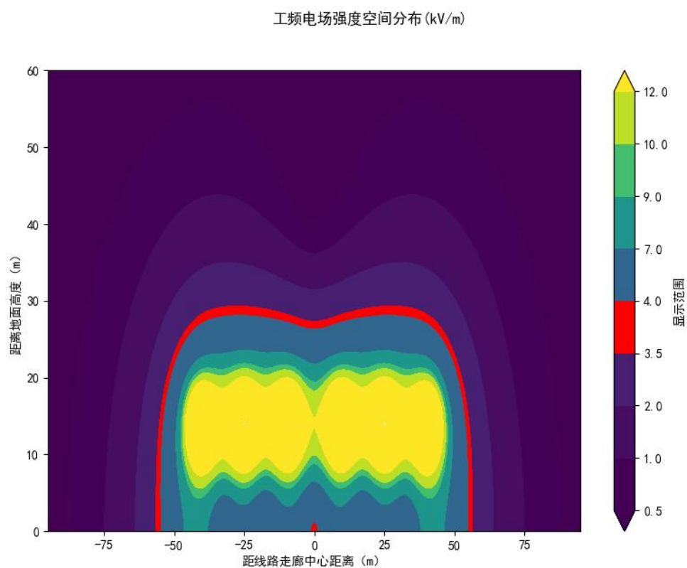
图 6-19 500kV 单回并行线路非居民区工频磁场等值线预测图
