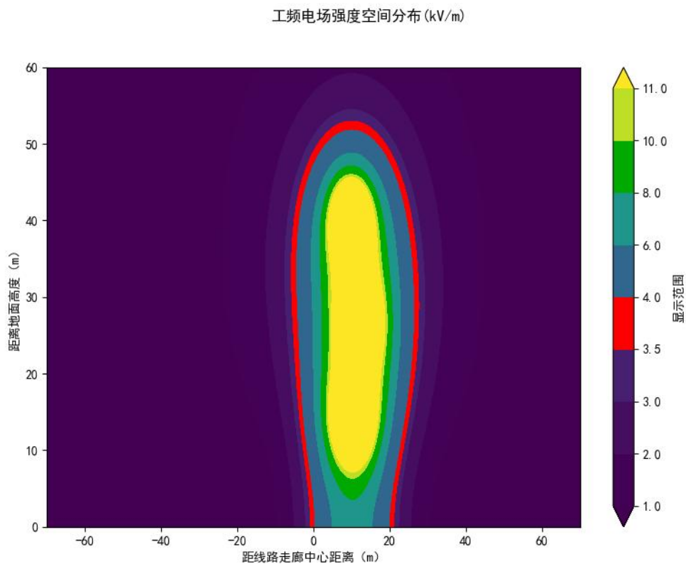
图 6-26 500kV 同塔双回单边挂线线路居民区工频电场等值线预测图
