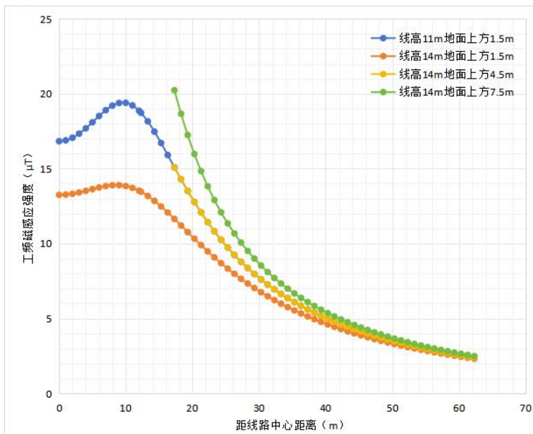
图 6-29 新建 500kV 同塔双回线路工频磁感应强度分布图
