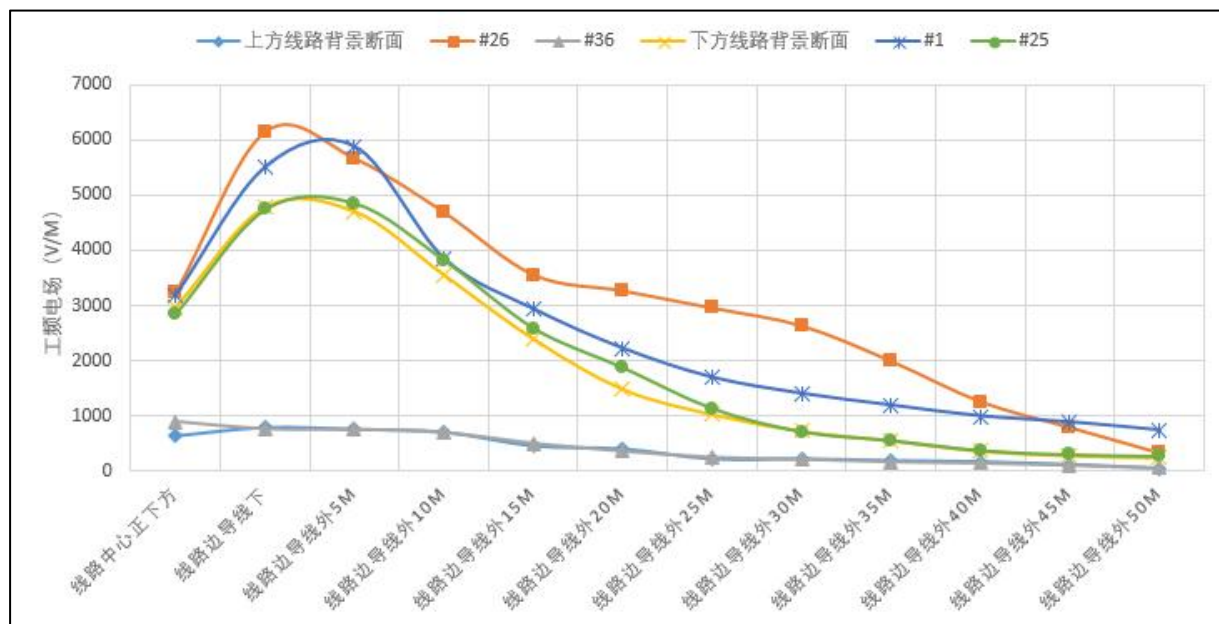
图 6-37 500kV 嵯螺 I 线和 500kV 嵯擎 I、II 线的部分断面监测数据示意图
