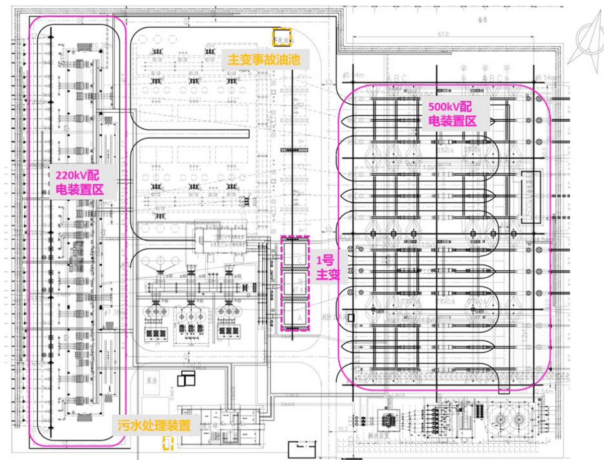
图 3-1 水场 500kV 变电站总平面布置图
