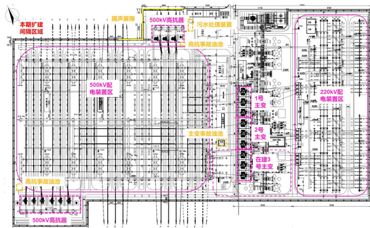
图 3-2 八河 500kV 变电站总平面布置图
