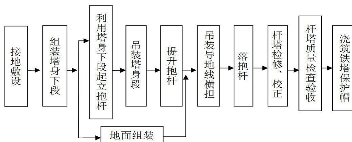
图 3-4 输电线路杆塔组立及接地工程施工流程图
