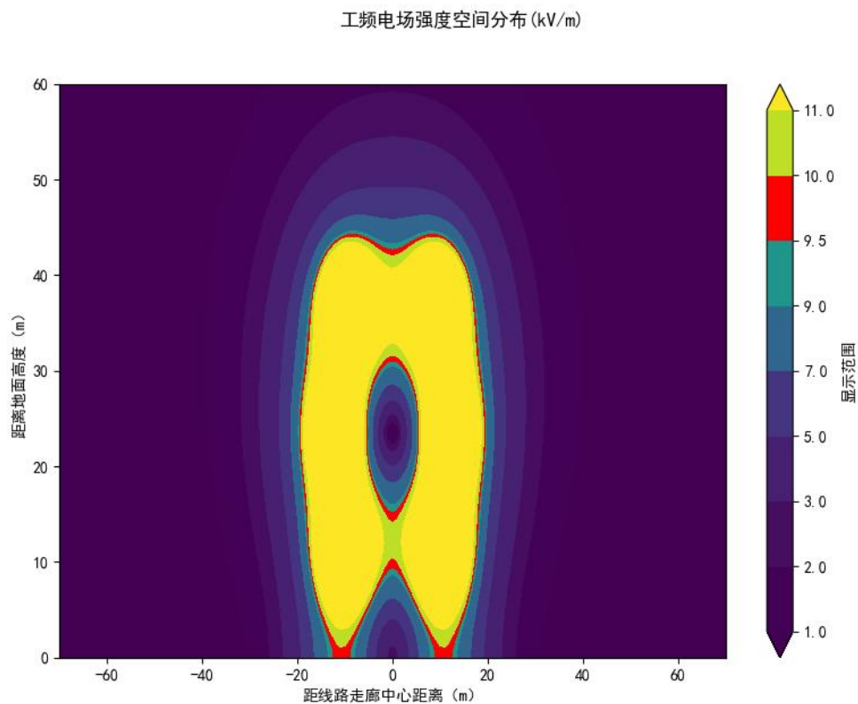
图 6-30 500kV 同塔双回线路非居民区工频电场等值线预测图
