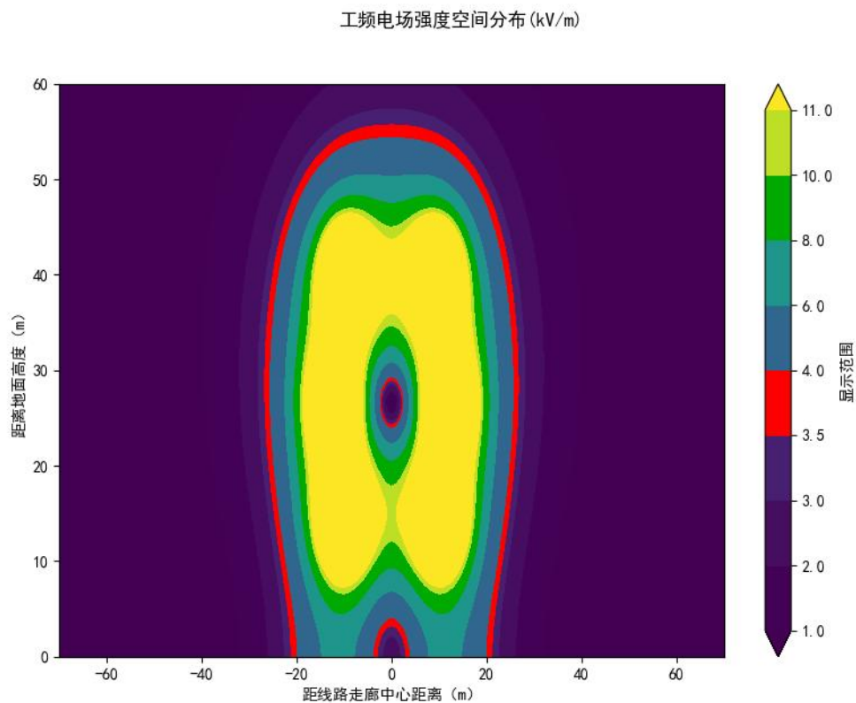
图 6-32 500kV 同塔双回线路居民区工频电场等值线预测图
