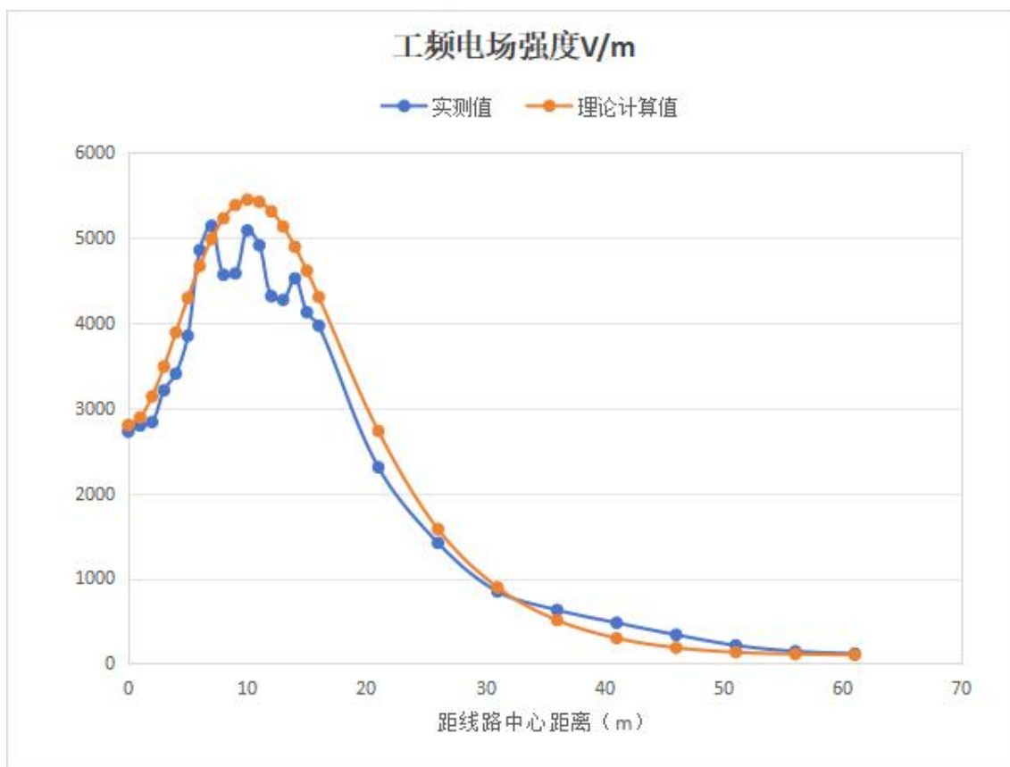
图 6-8 500kV 雁船 I、II 回工频电场强度类比监测结果与理论计算结果示意图
