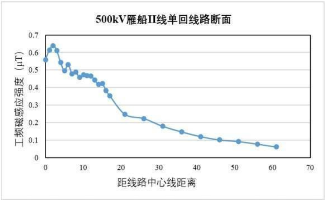
图 6-4 500kV 雁船 II 线单回线路断面工频电场强度、磁感应强度变化趋势图
