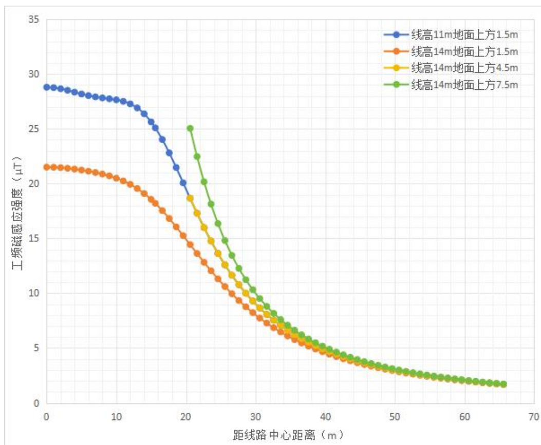
图 6-11 新建 500kV 单回线路工频磁感应强度分布图
