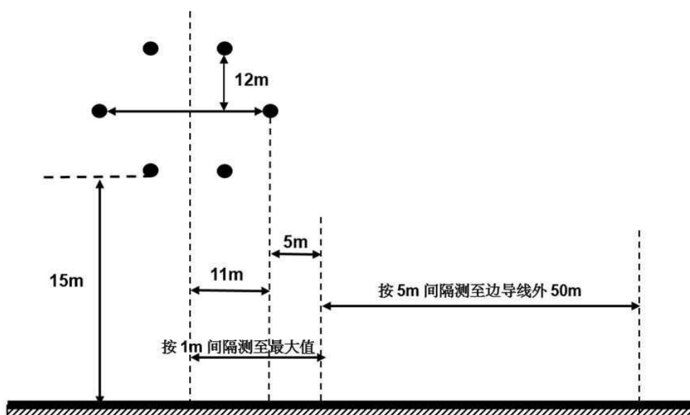
图 6-3 500kV 雁船 I 回线、雁船 II 回线#027~#028 同塔双回线路段电磁环境监测断面示意图
