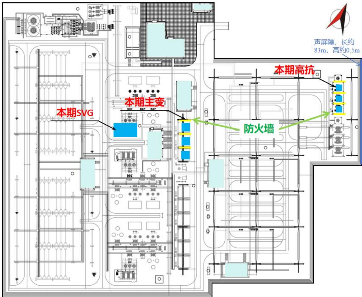
图 6-43 变电站围墙加装隔声屏障示意图
