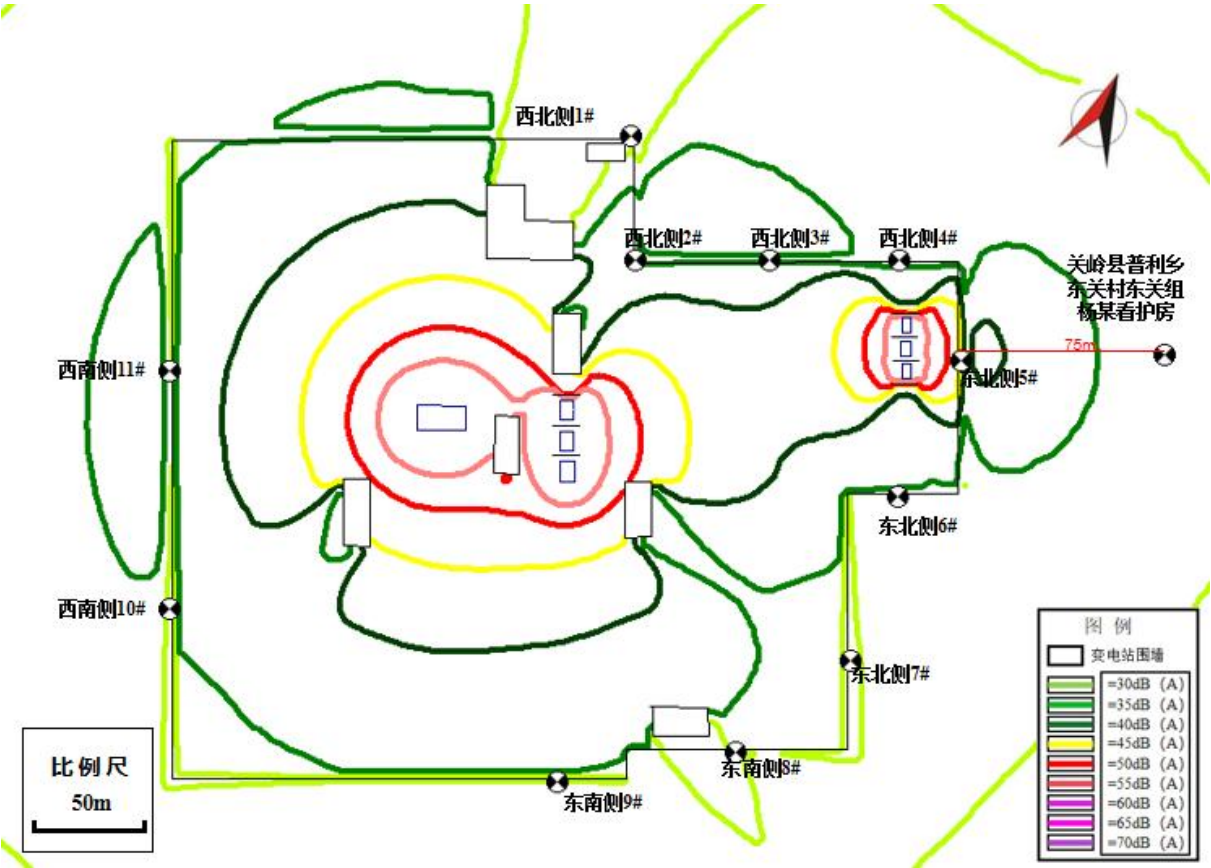
图 6-44 关岭 500kV 变电站设置隔声屏障后本期噪声贡献值等值线分布图（预测点高 1.2m）
