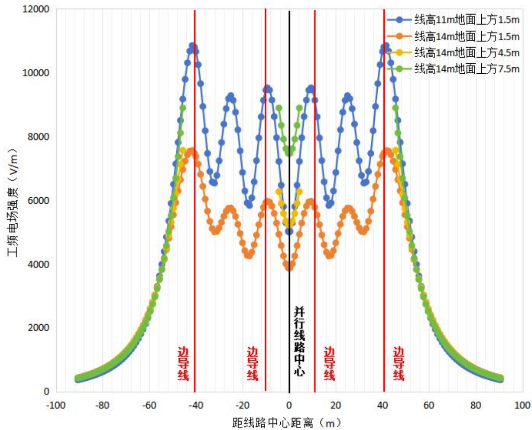
图 6-16 新建 500kV 单回并行线路工频电场强度分布图
