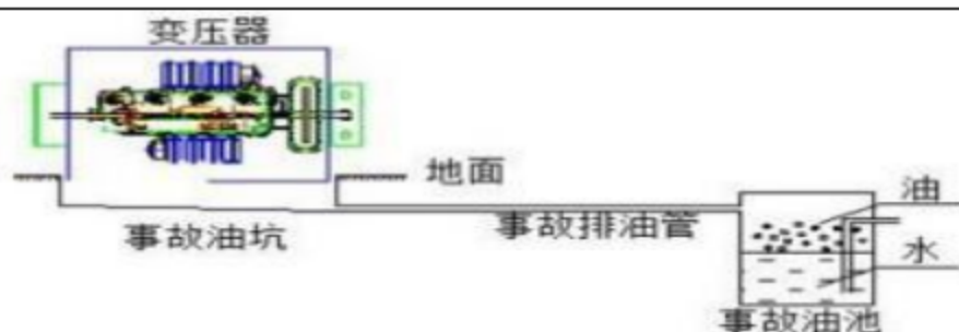
图6.5-1 事故油池处置原理示意图
