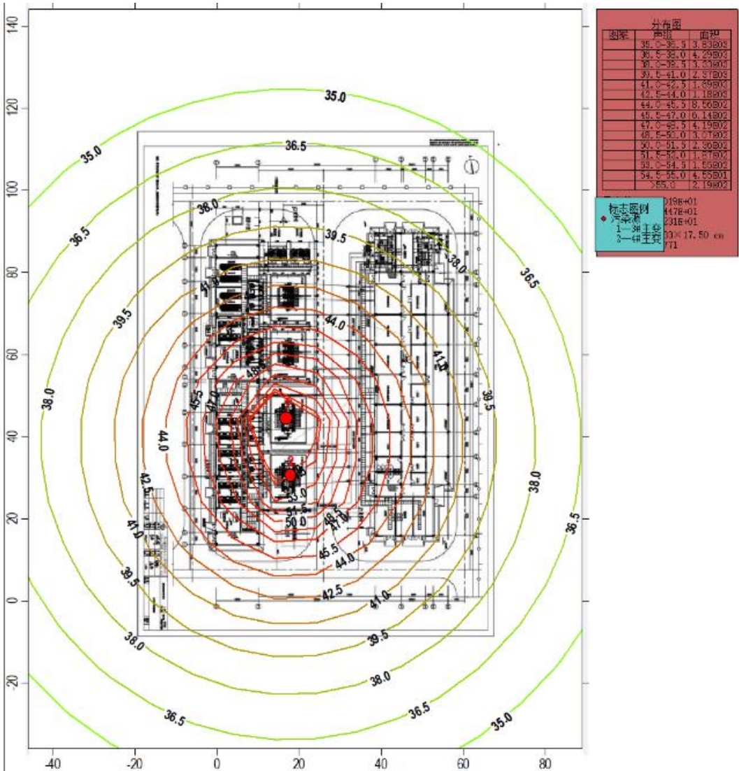
图4-3 噪声贡献值等声级线图
