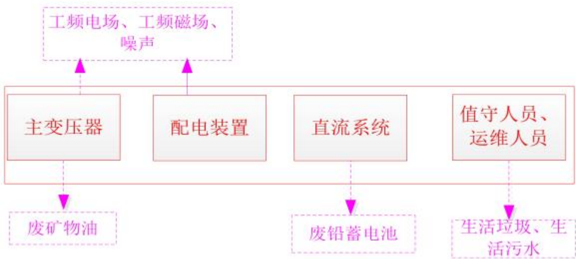
图 4-2 变电站运营期产污节点图
