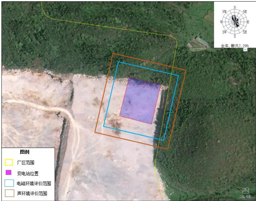
图 3-1 盛屯 220kV 变电站评价范围图
