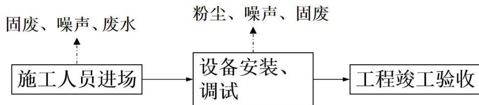
图 4-1 本次扩建项目施工期工艺流程及产污位置示意图
