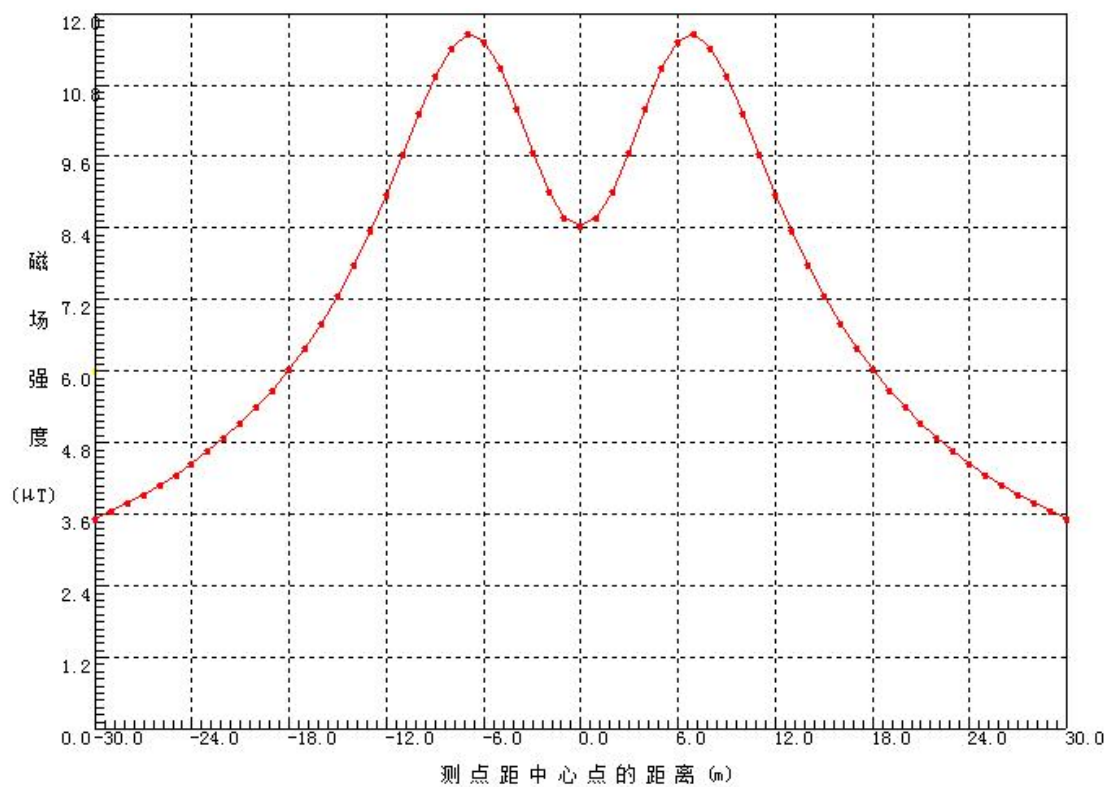
图 5-6 导线对地最小垂直距离为 7.5m 时线下工频磁场强度分布曲线
