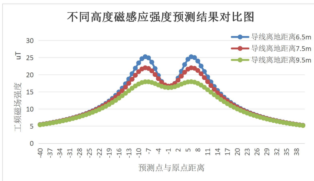
图 5-8 不同高度线下工频电场强度分布曲线对比图
