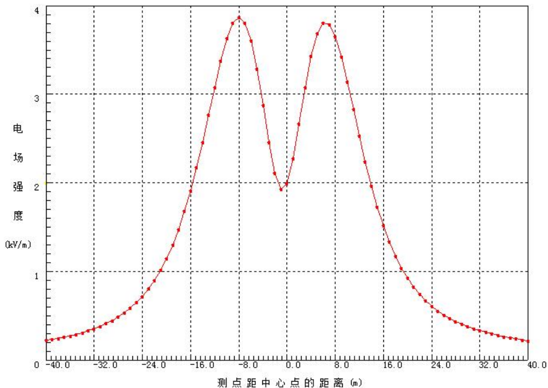
图 5-3 导线对地最小距离为 9.5m 时线下工频电场强度分布曲线
