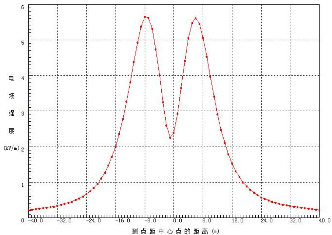
图 5-2 导线对地最小距离为 7.5m 时线下工频电场强度分布曲线
