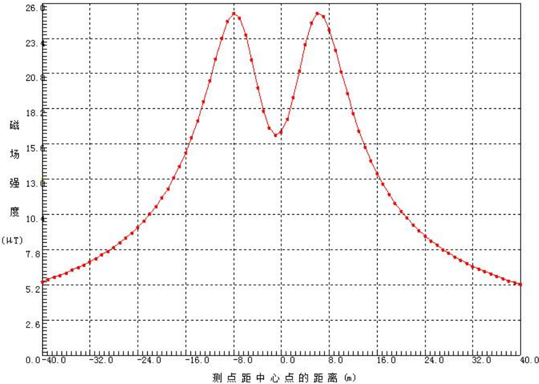
图 5-5 导线对地最小垂直距离为 6.5m 时线下工频磁场强度分布曲线
