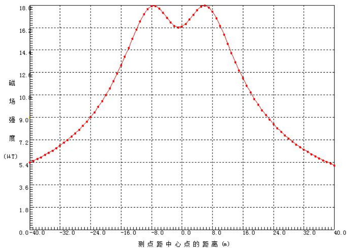
图 5-7 导线对地最小垂直距离为 9.5m 时线下工频磁场强度分布曲线
