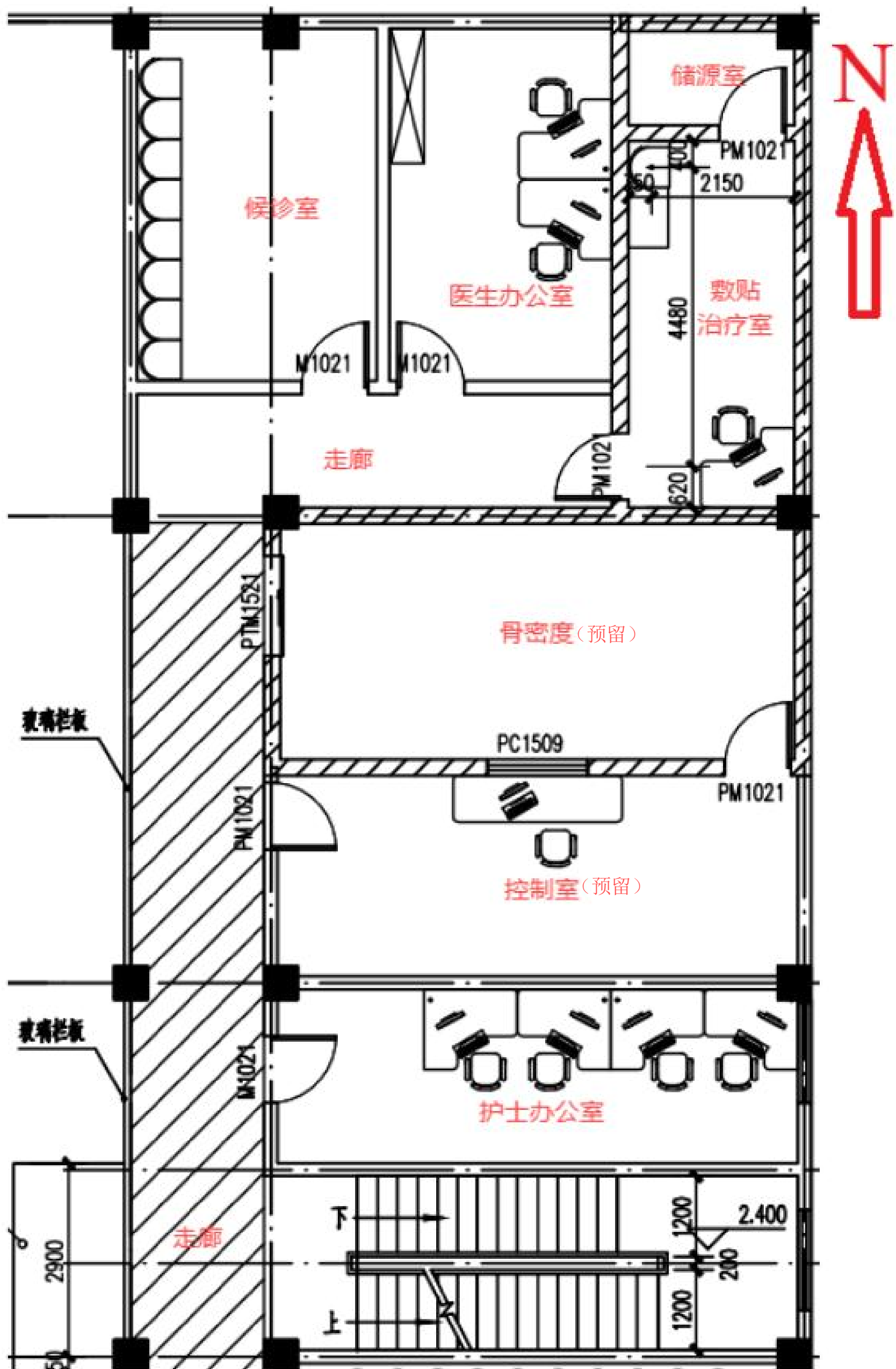
附图四：核医学科二层北区敷贴治疗室及预留骨密度室平面布置图
