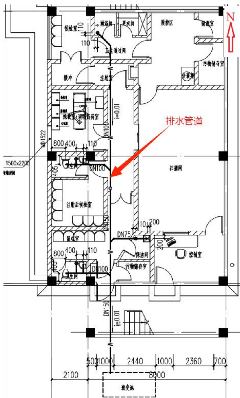
图 10-5 核医学科污水管道布置图
