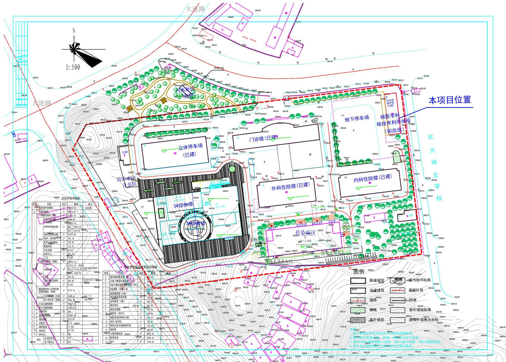
附图一：六盘水市钟山区人民医院总平面布置图
