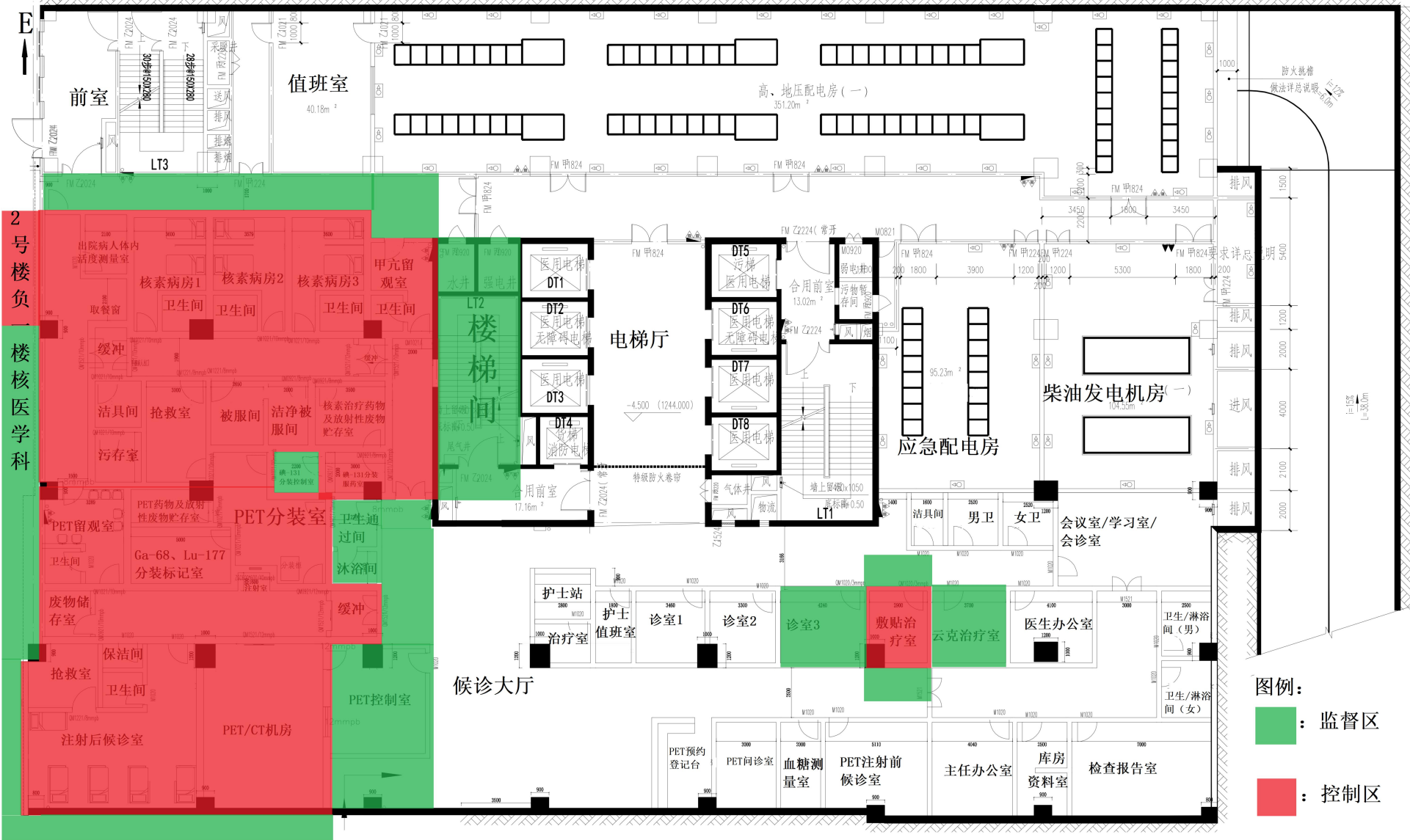
附图 7：3 号楼负一楼核医学科分区图
